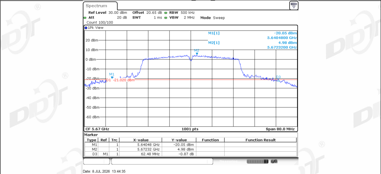
11N40MIMO_Ant2_5670
