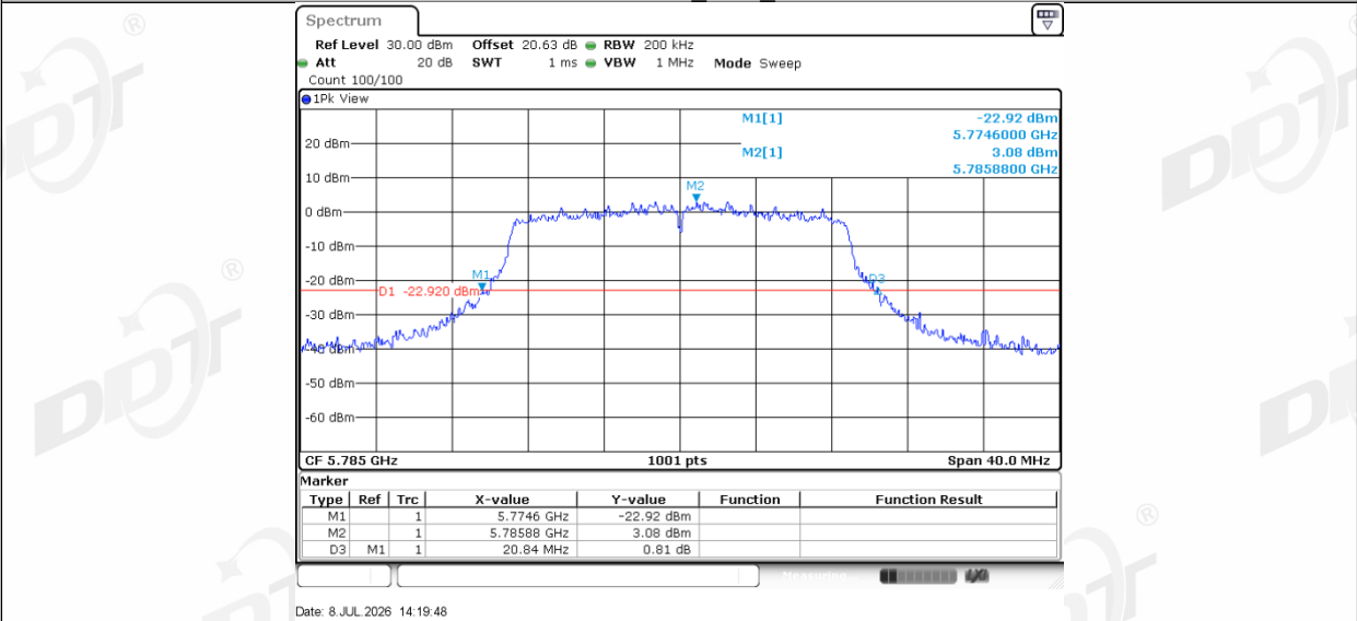
11AC20MIMO_Ant2_5785
