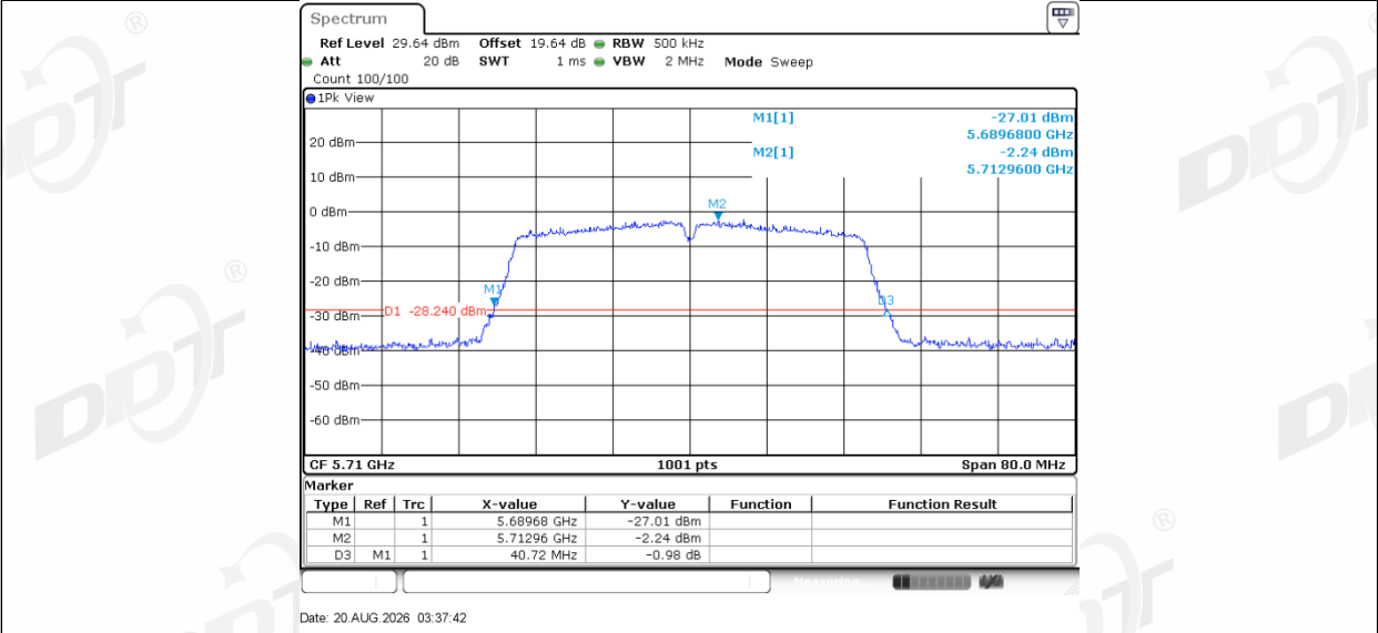
11AC40MIMO_Ant2_5710
