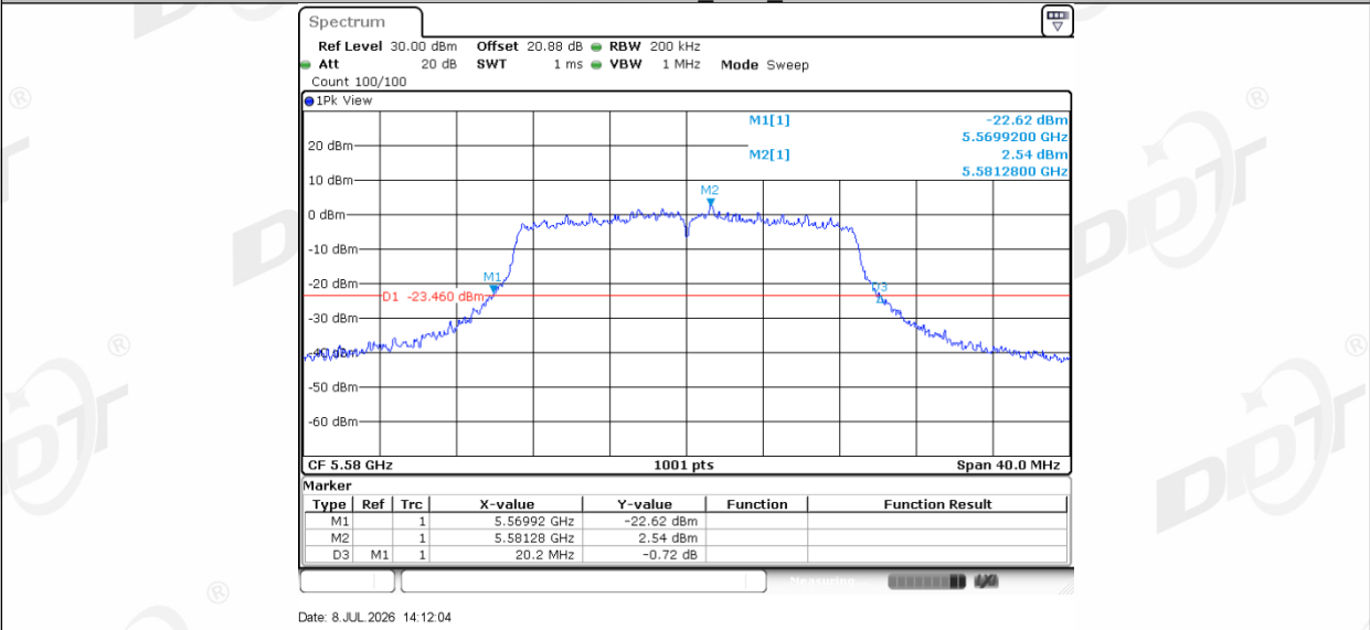
11AC20MIMO_Ant2_5580
