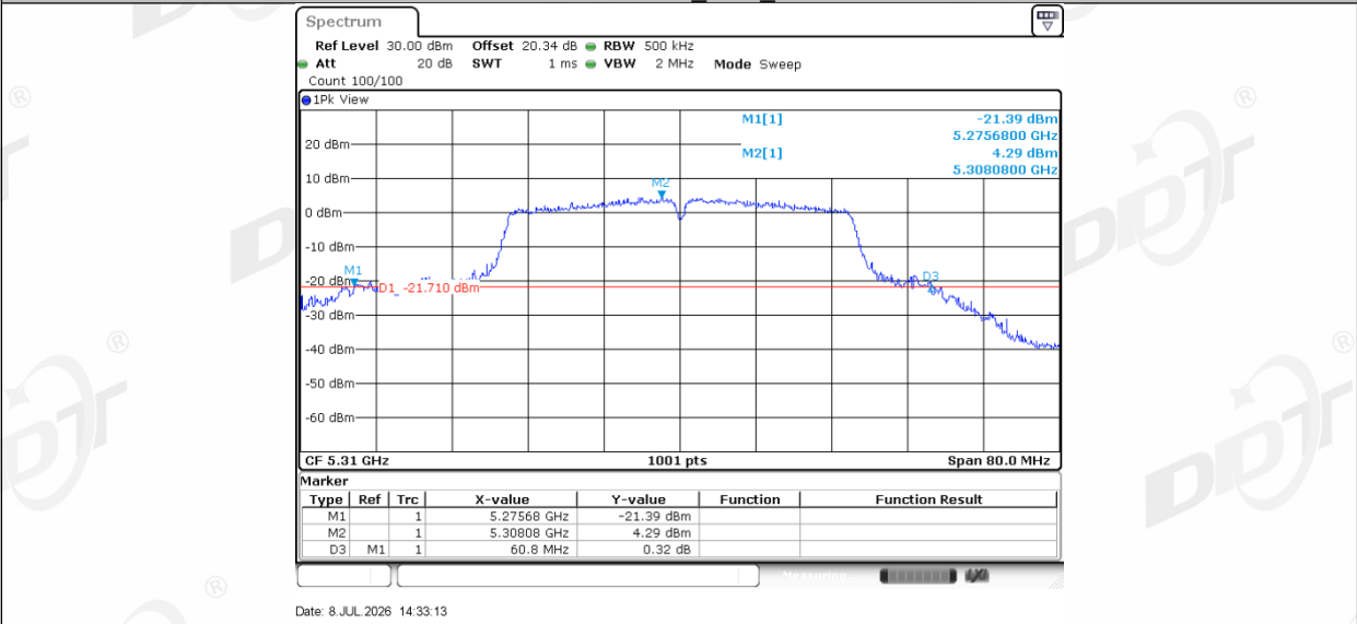
11AC40MIMO_Ant2_5310
