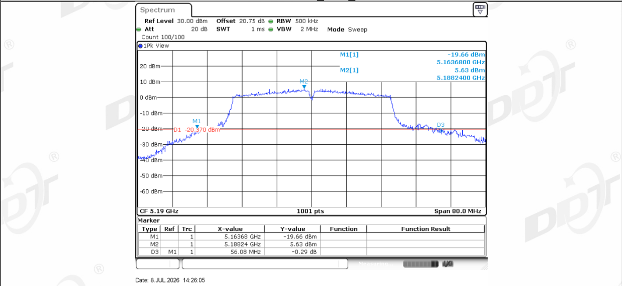
11AC40MIMO_Ant2_5190
