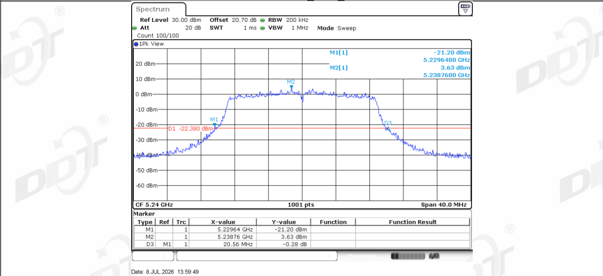
11AC20MIMO_Ant2_5240
