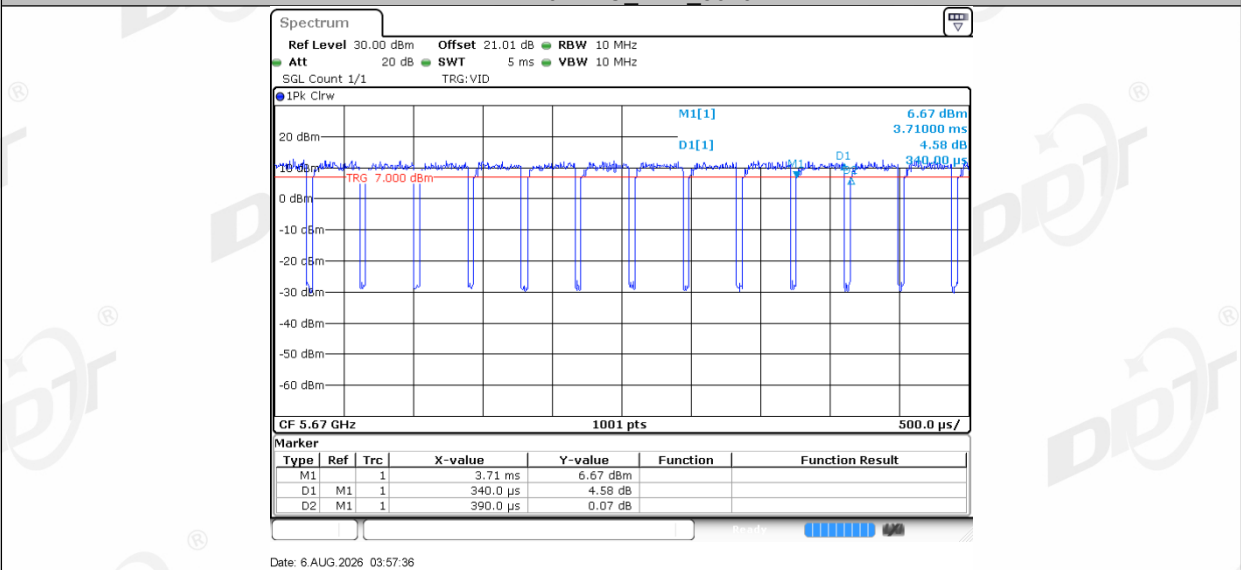
11N40MIMO_Ant2_5670
