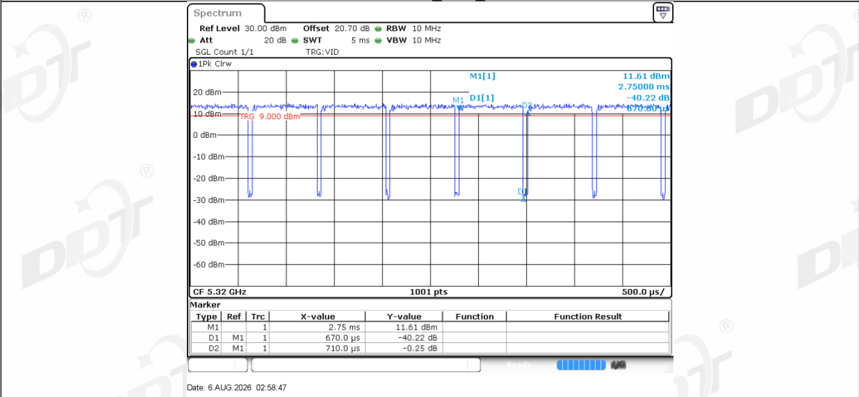
11N20MIMO_Ant2_5320
