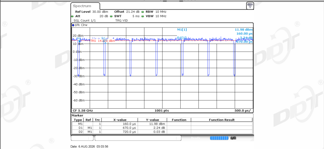
11N20MIMO_Ant2_5580
