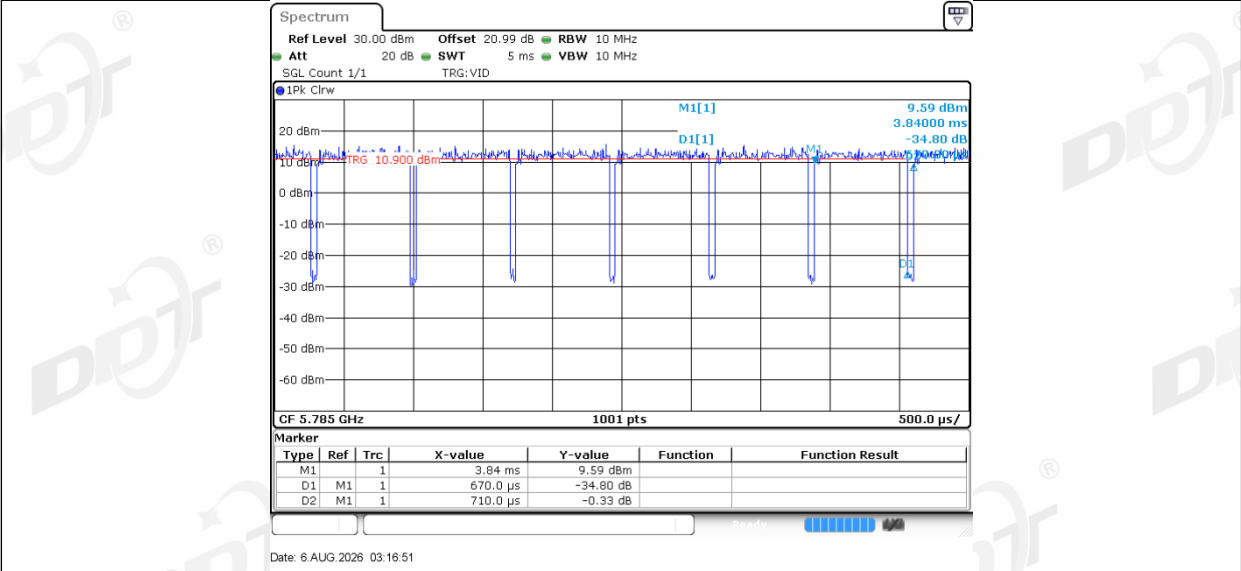
11N20MIMO_Ant2_5785
