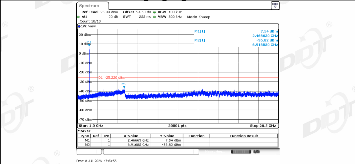
11G_Ant2_2462
