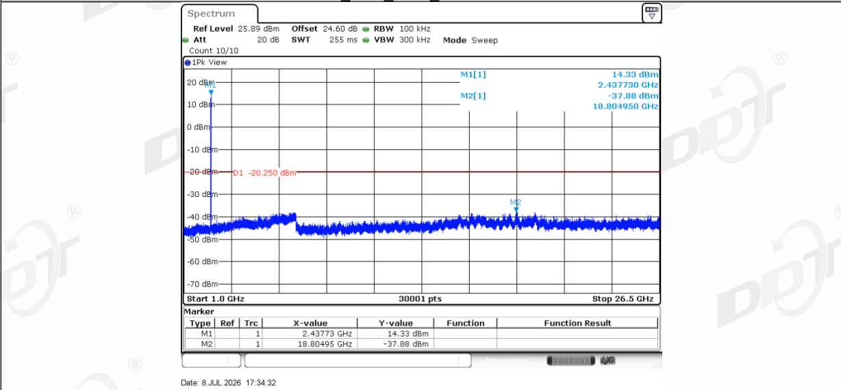
11B_Ant2_2437
