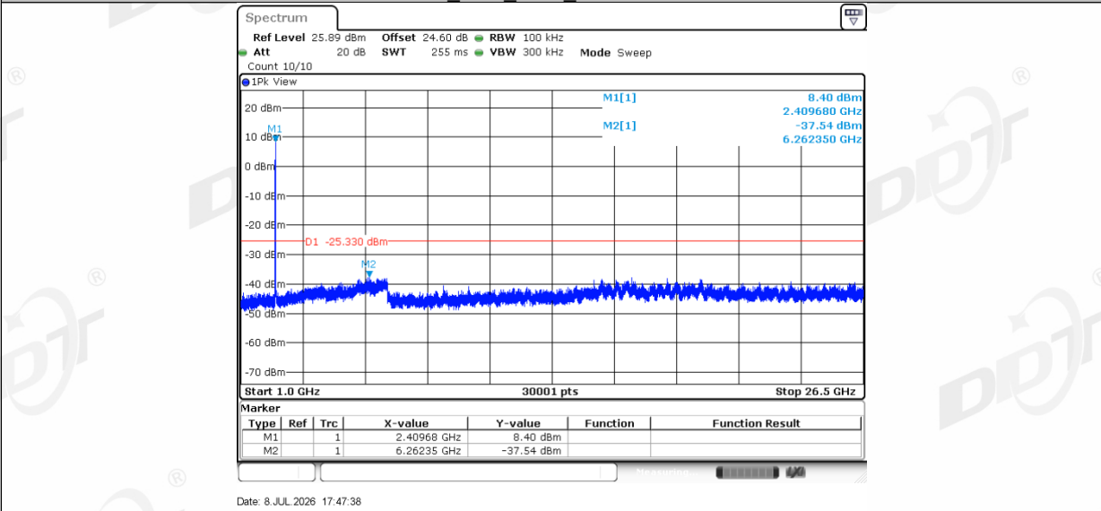
11G_Ant2_2412
