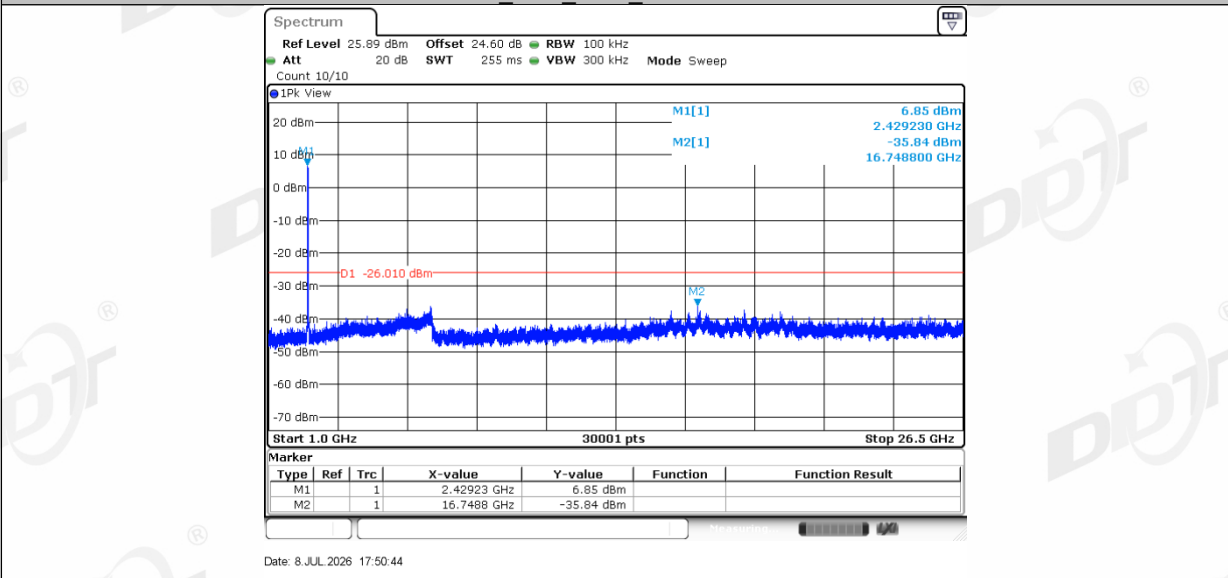
11G_Ant2_2437
