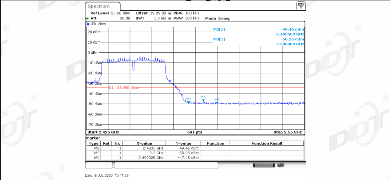
11N40MIMO_Ant2_High_2452
