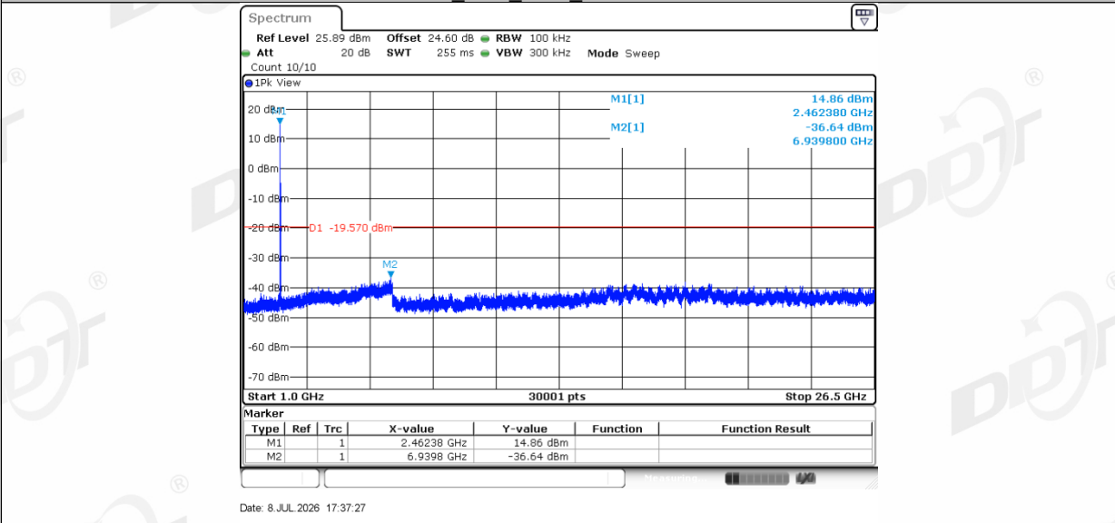
11B_Ant2_2462
