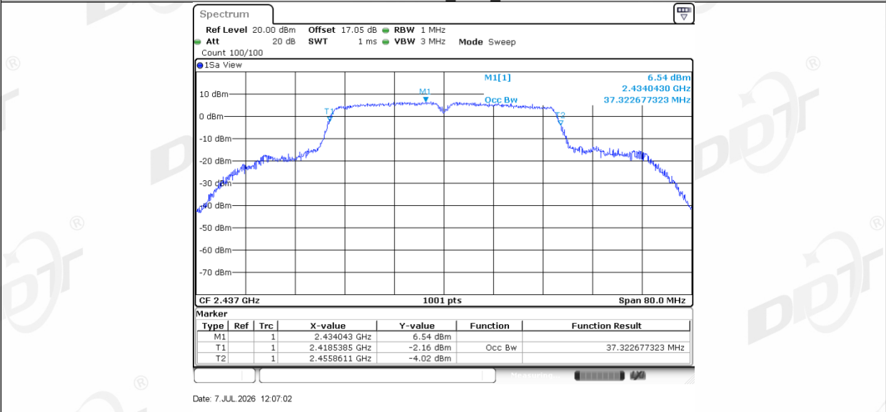
11N40MIMO_Ant2_2437
