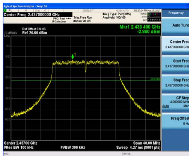
802.11n(HT20) CH06
