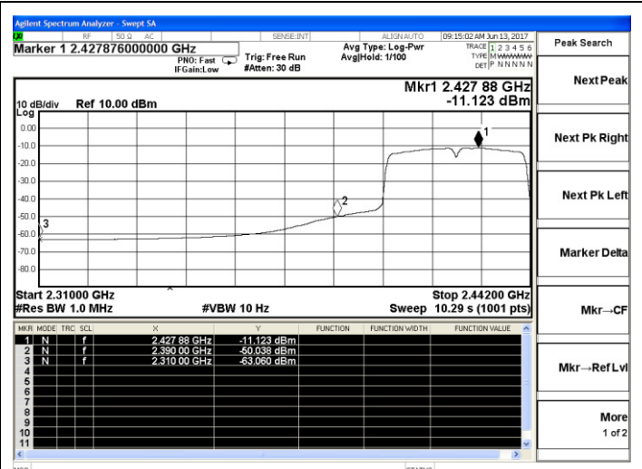
802.11n-HT40 Low channel(Average)
