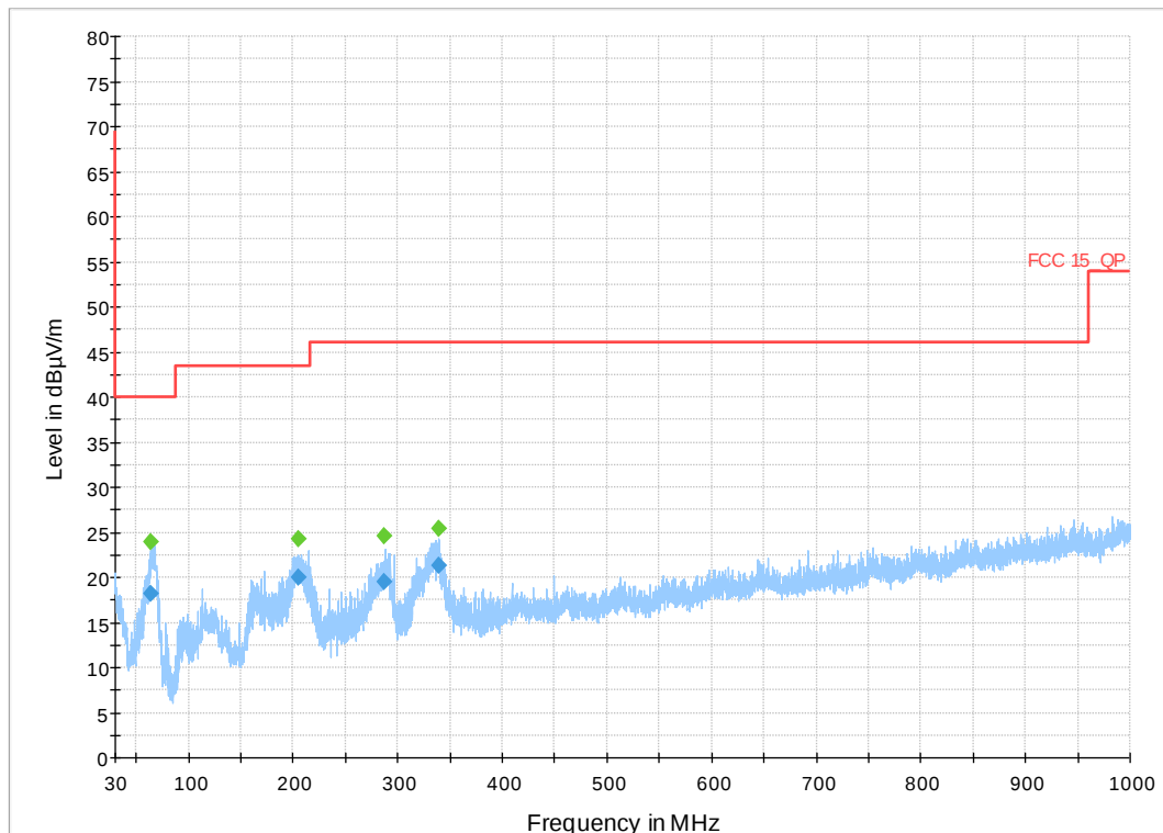
Plot 35. 30MHz-1000MHz, 1Mbps, 2402MHz
