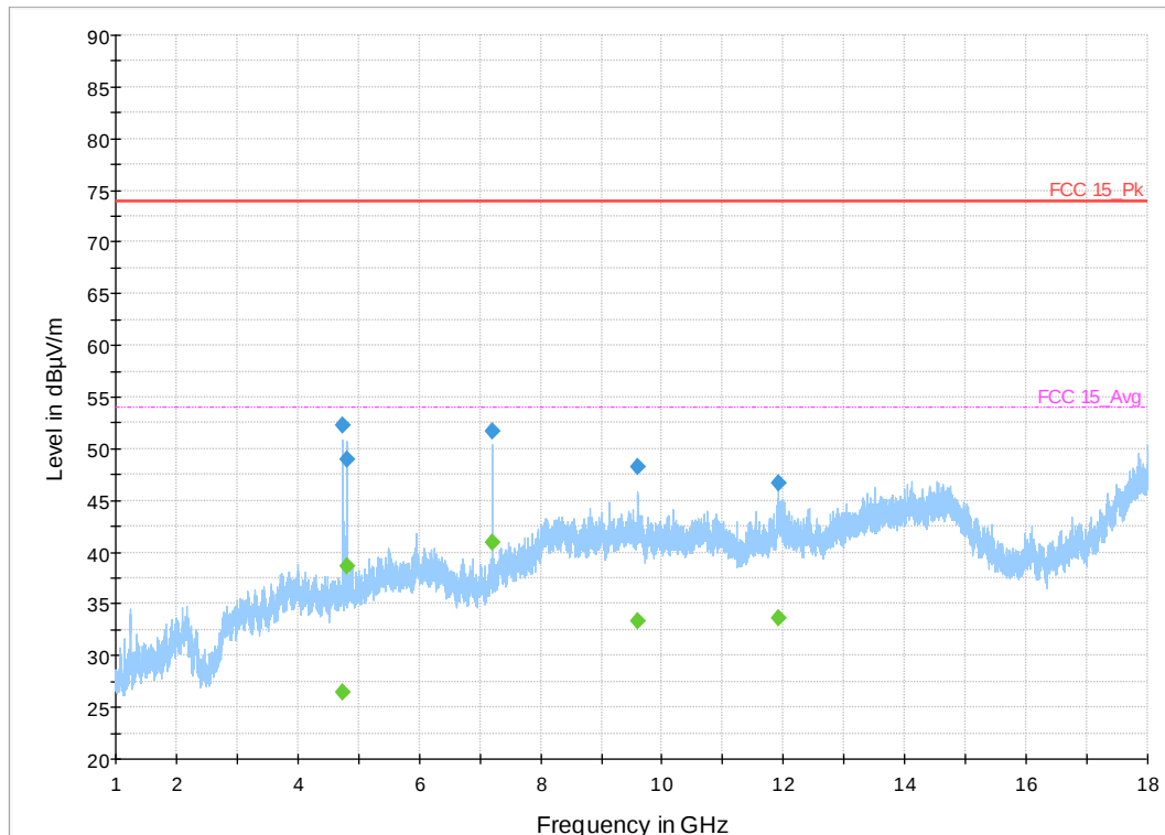
Plot 38. 1-18GHz, 1Mbps, 2402MHz
