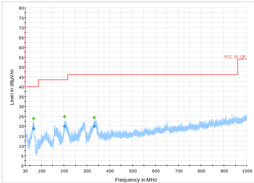
Plot 36. 30MHz-1000MHz, 1Mbps, 2440MHz
