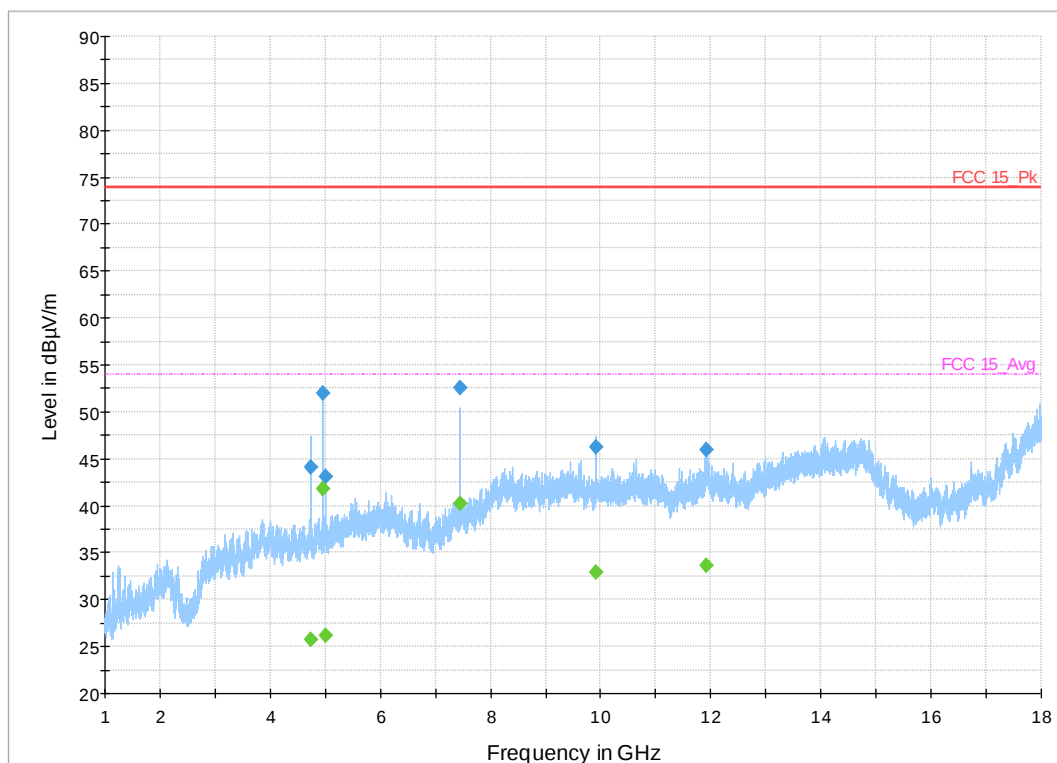
Plot 40. 1-18GHz, 1Mbps, 2480MHz
