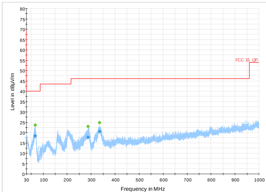
Plot 37. 30-1000MHz, 1Mbps, 2480MHz
