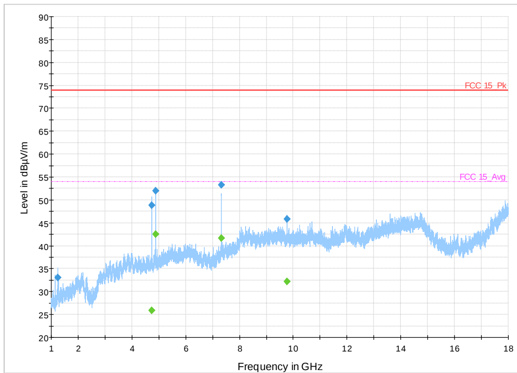
Plot 39. 1-18GHz, 1Mbps, 2440MHz
