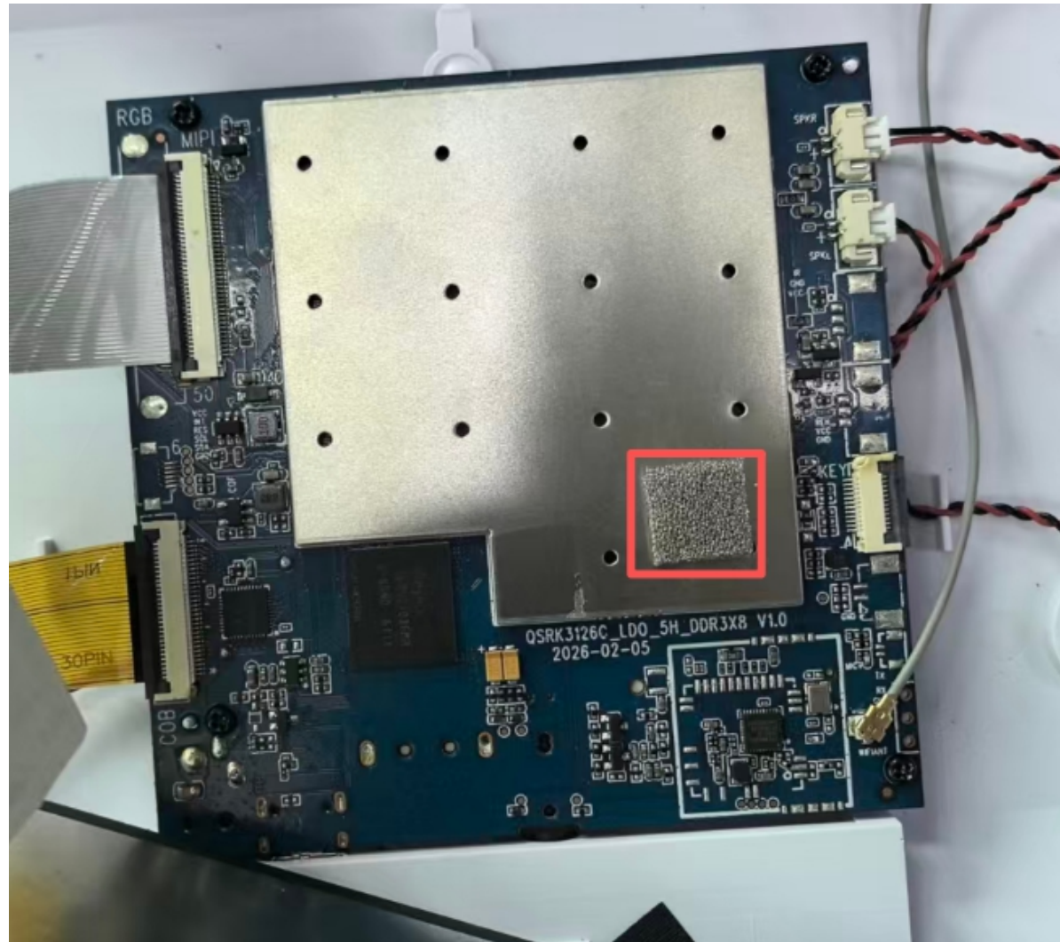
主板屏蔽盖贴导电海绵跟屏接地
