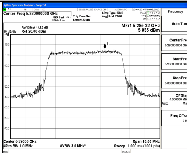
11AX20MIMO Ant2 5280
