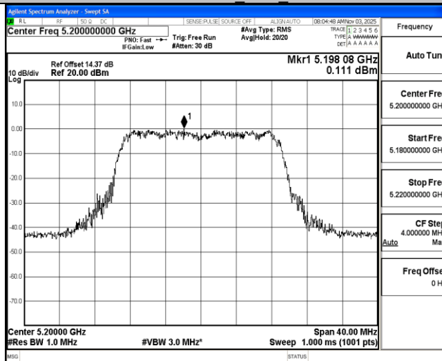
11AC20MIMO_Ant2_5200
