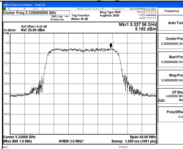
11AX20MIMO Ant2 5320
