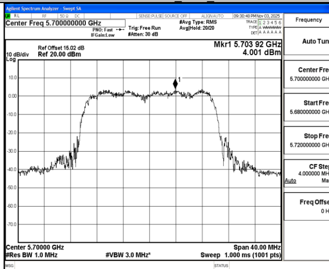
11AX20MIMO Ant2 5700
