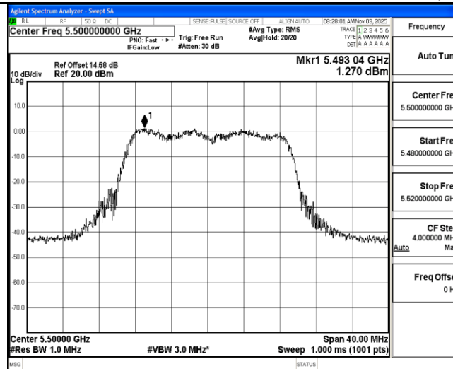
11AC20MIMO_Ant2_5500
