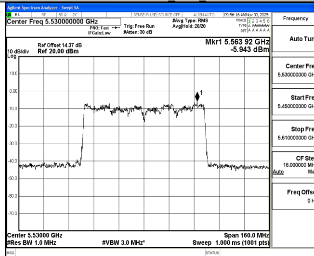
11AC80MIMO_Ant2_5530
