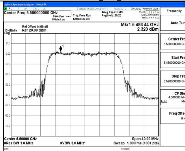
11AX20MIMO Ant2 5500
