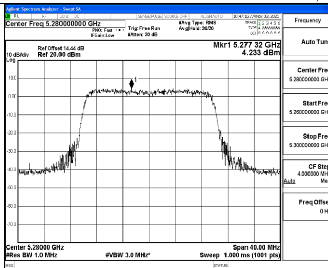
11AX20MIMO Ant2 5280
