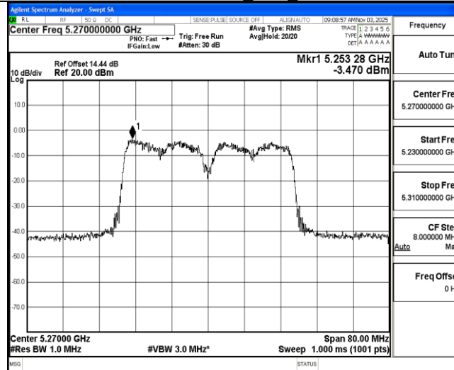
11AC40MIMO_Ant2_5270
