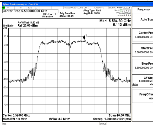
11AX20MIMO Ant2 5580
