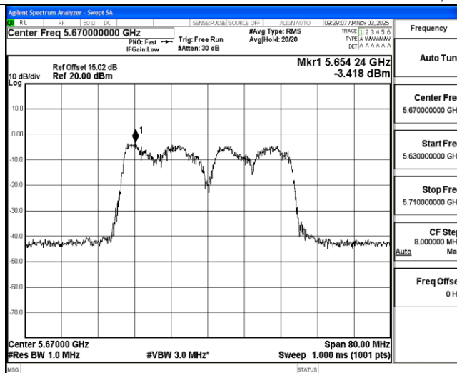
11AC40MIMO_Ant2_5670
