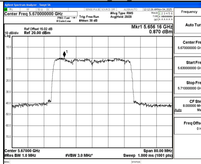
11AX40MIMO_Ant2_5670
