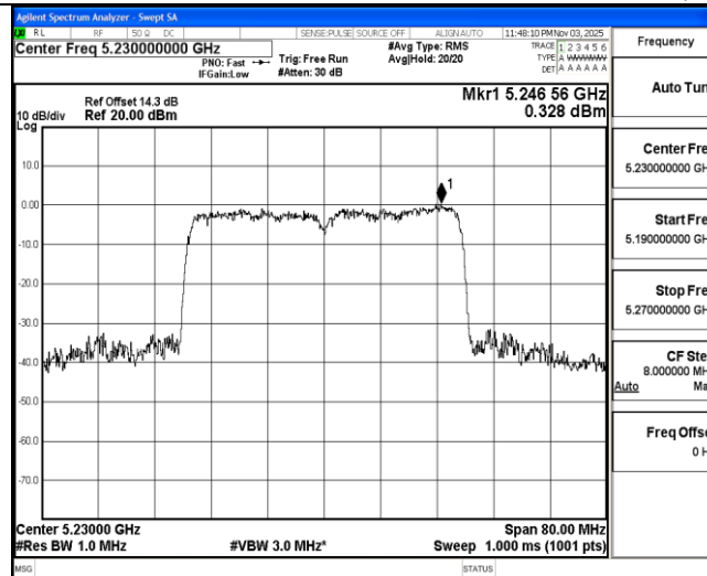
11AX40MIMO Ant2 5230
