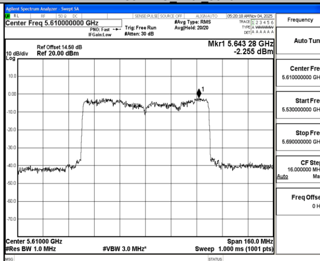
11AX80MIMO_Ant1_5610
