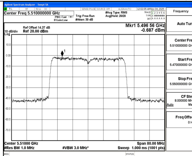
11AX40MIMO Ant2 5510
