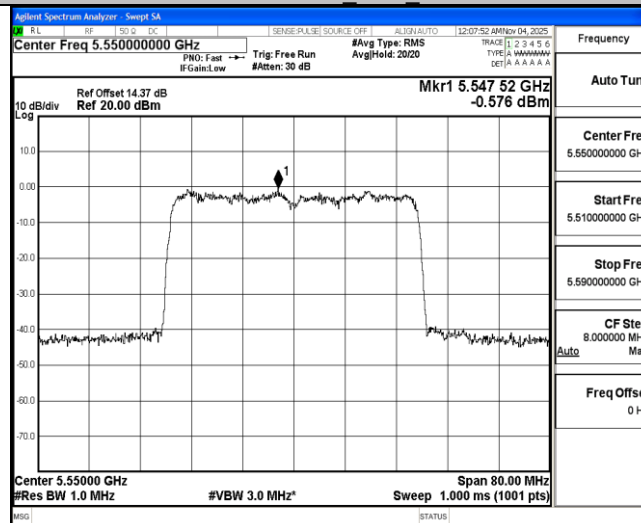
11AX40MIMO Ant2 5550
