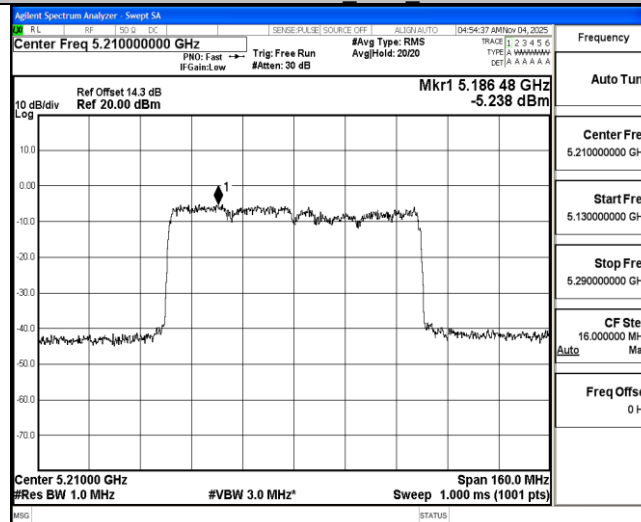
11AX80MIMO_Ant2_5210
