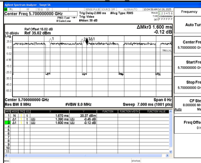
11N20MIMO Ant2 5700
