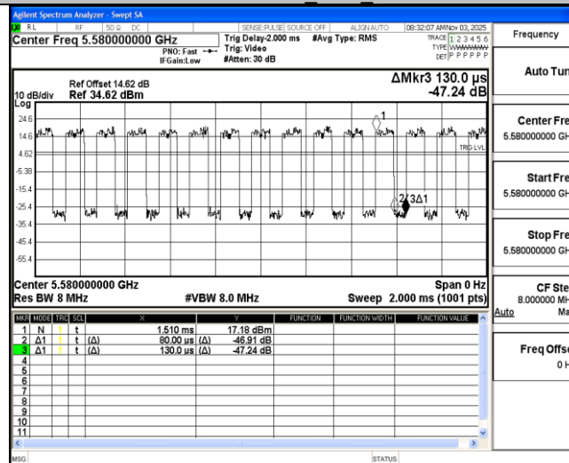
11AC20MIMO_Ant2_5580
