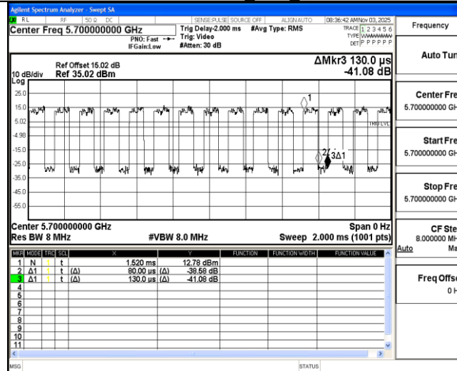
11AC20MIMO_Ant2_5700
