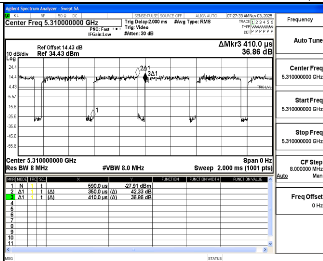
11N40MIMO Ant2 5310
