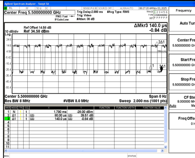
11AC20MIMO_Ant2_5500
