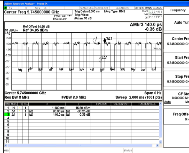
11AC20MIMO_Ant2_5745
