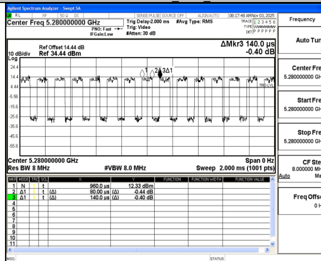
11AC20MIMO_Ant2_5280
