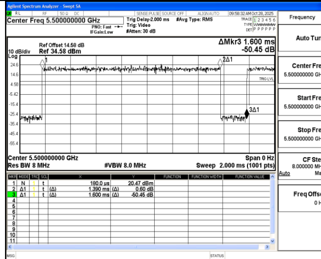
11N20MIMO Ant2 5500
