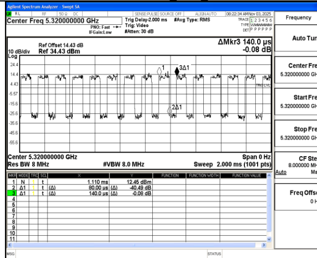
11AC20MIMO_Ant2_5320
