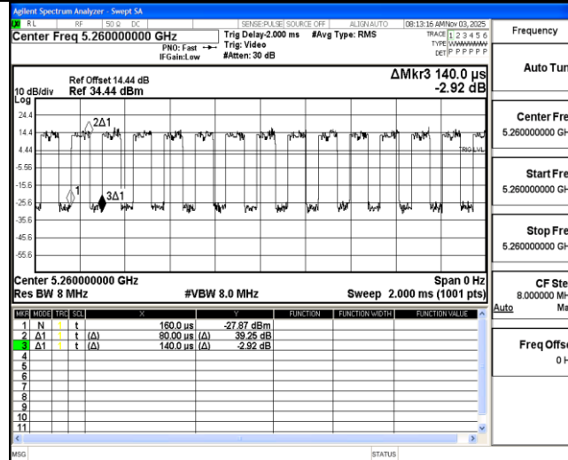
11AC20MIMO_Ant2_5260
