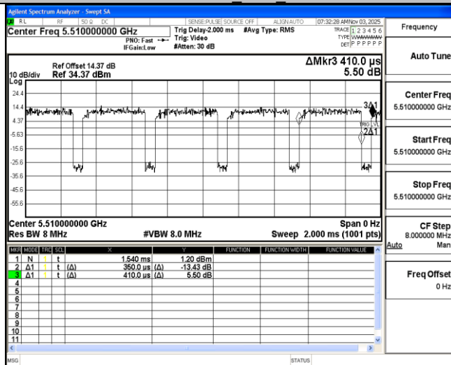
11N40MIMO Ant2 5510
