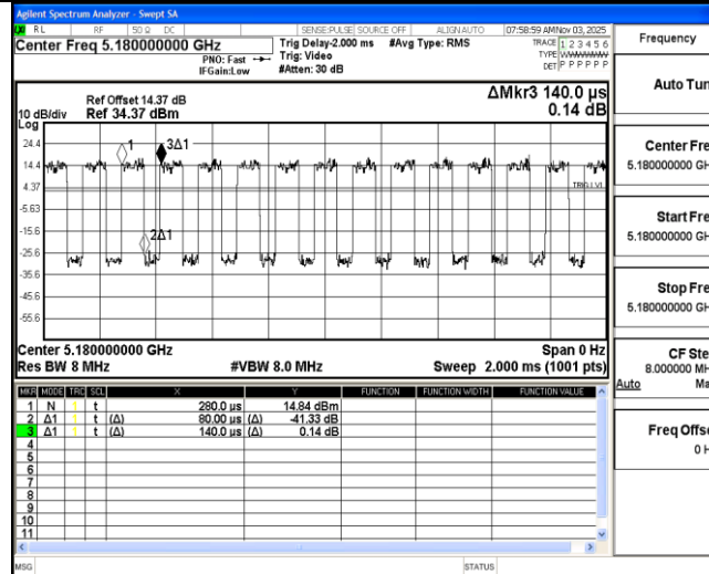
11AC20MIMO_Ant2_5180
