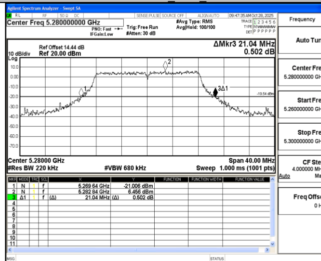
11N20MIMO Ant2 5280
