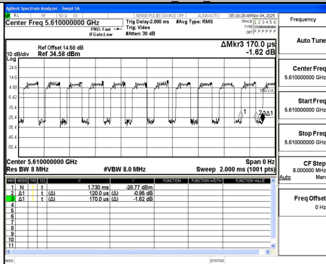
11AX80MIMO_Ant2_5610
