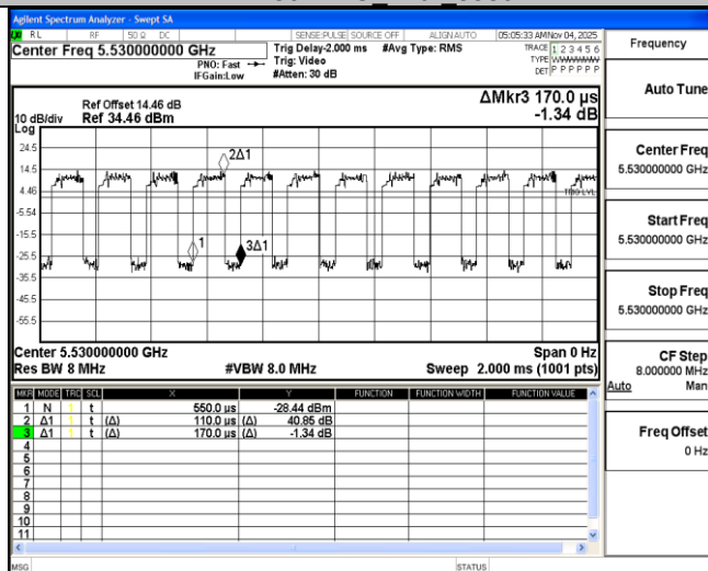
11AX80MIMO_Ant2_5530
