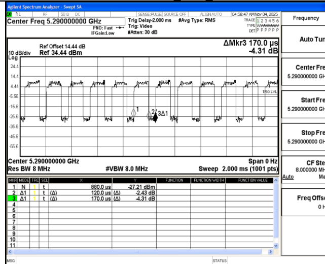
11AX80MIMO_Ant2_5290
