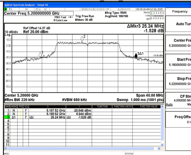
11N20MIMO Ant2 5200
