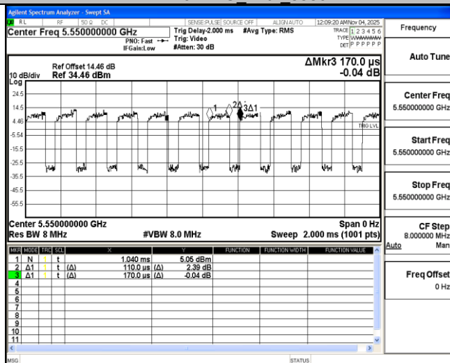
11AX40MIMO Ant2 5550
