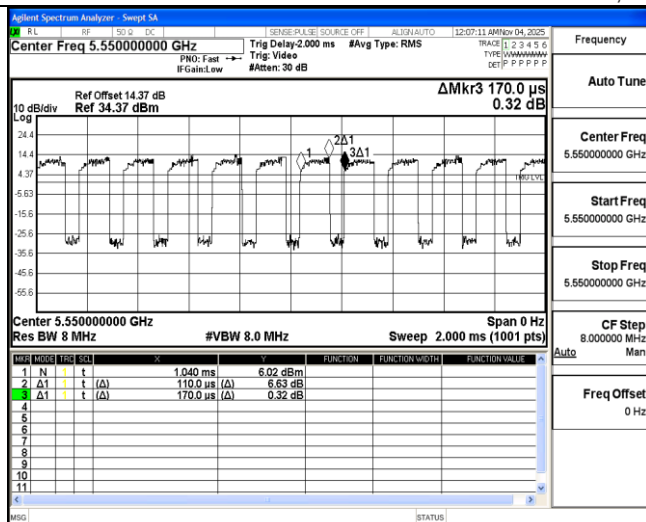
11AX40MIMO Ant2 5550
