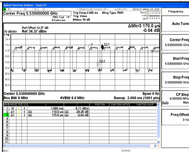
11AX80MIMO_Ant2_5530
