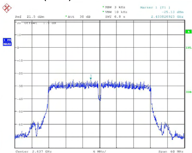
802.11n(HT40) 2437MHz
