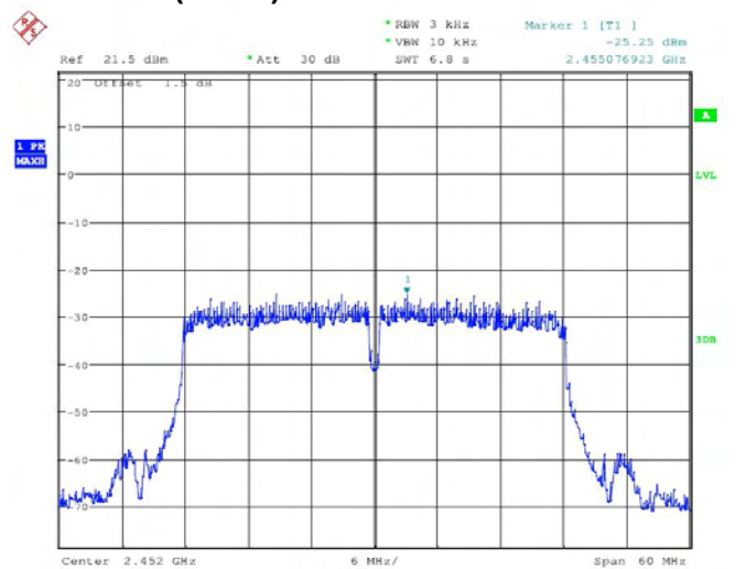
802.11n(HT40) 2452MHz
