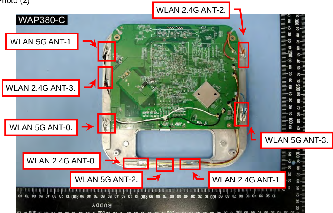
EUT Photo (2)
