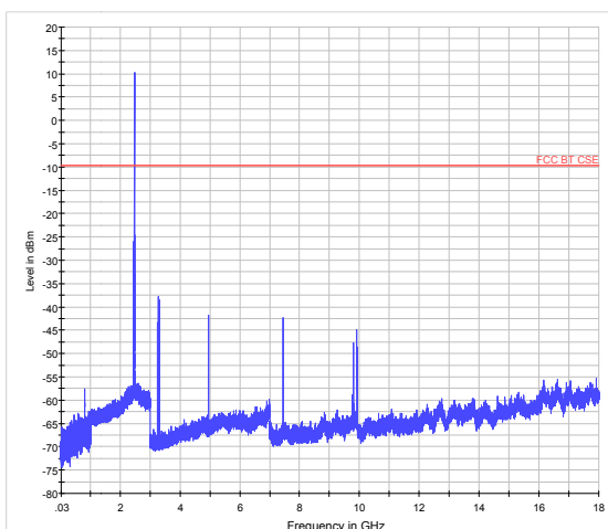
EDR - CH78 30MHz to 18GHz
