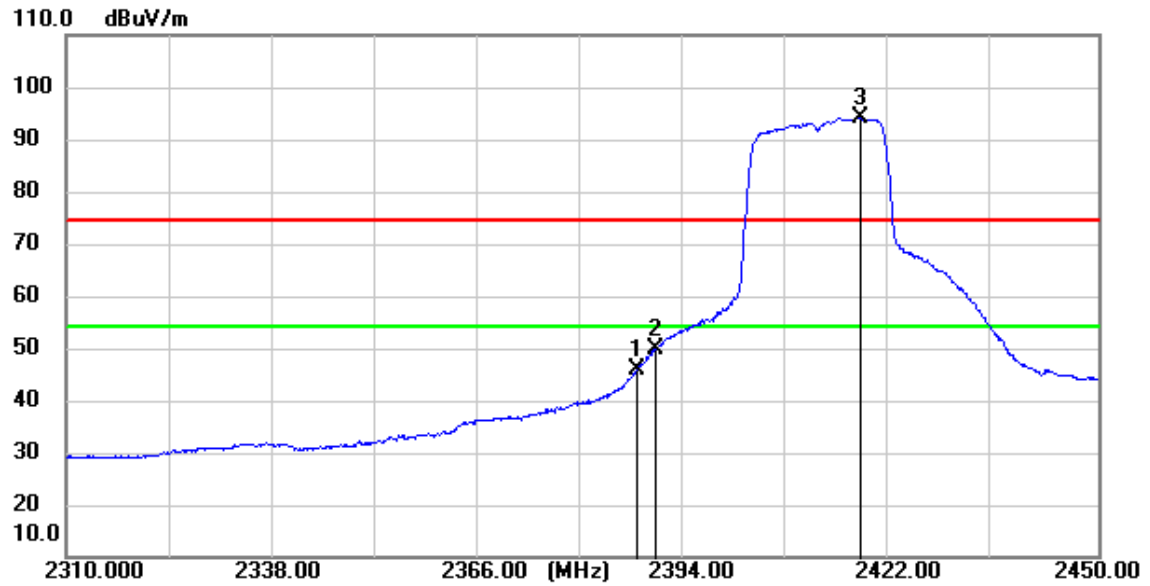
11n(HT20)_TX_CH_01_Horizontal_Average
