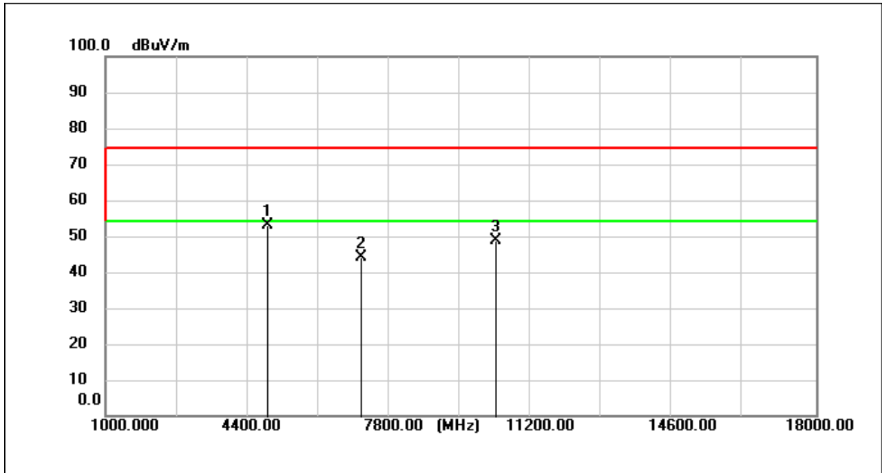
11b_TX_CH_06_Vertical
