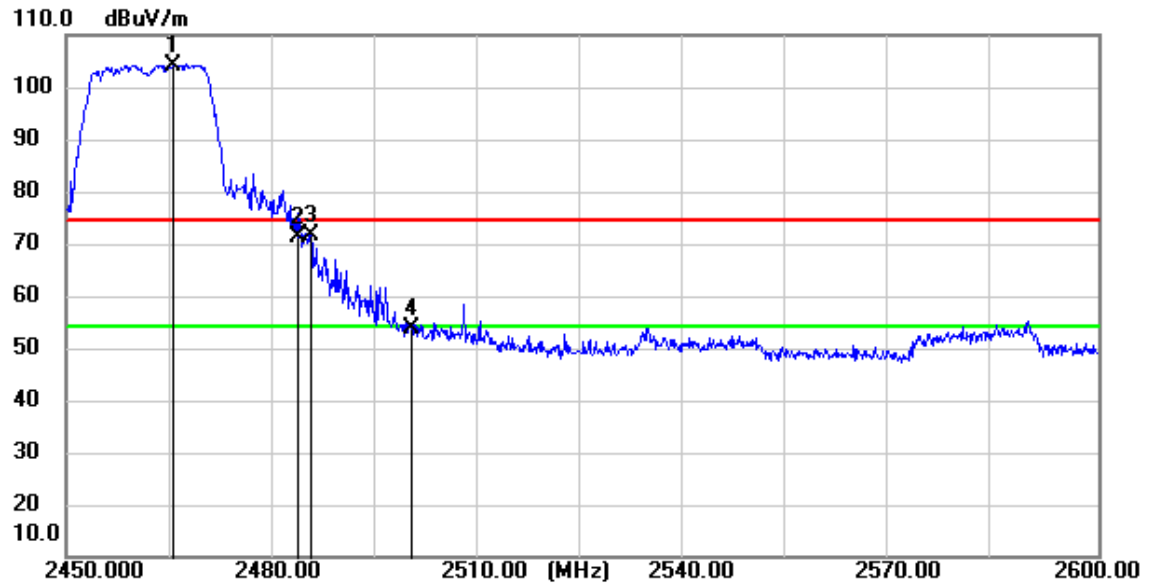
11n(HT20)_TX_CH_11_Horizontal_Peak
