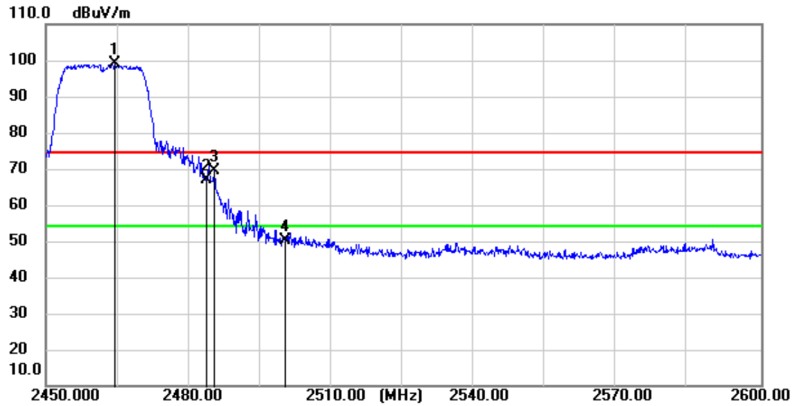
11n(HT20)_TX_CH_11_Vertical_Peak
