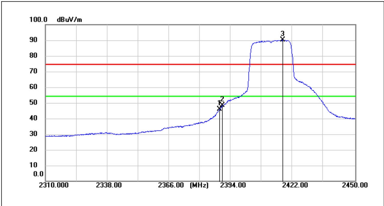
11n(HT20)_TX_CH_01_Vertical_Average
