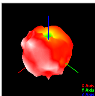
5.35GHz
