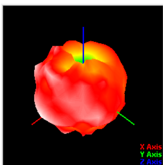
5.15GHz
