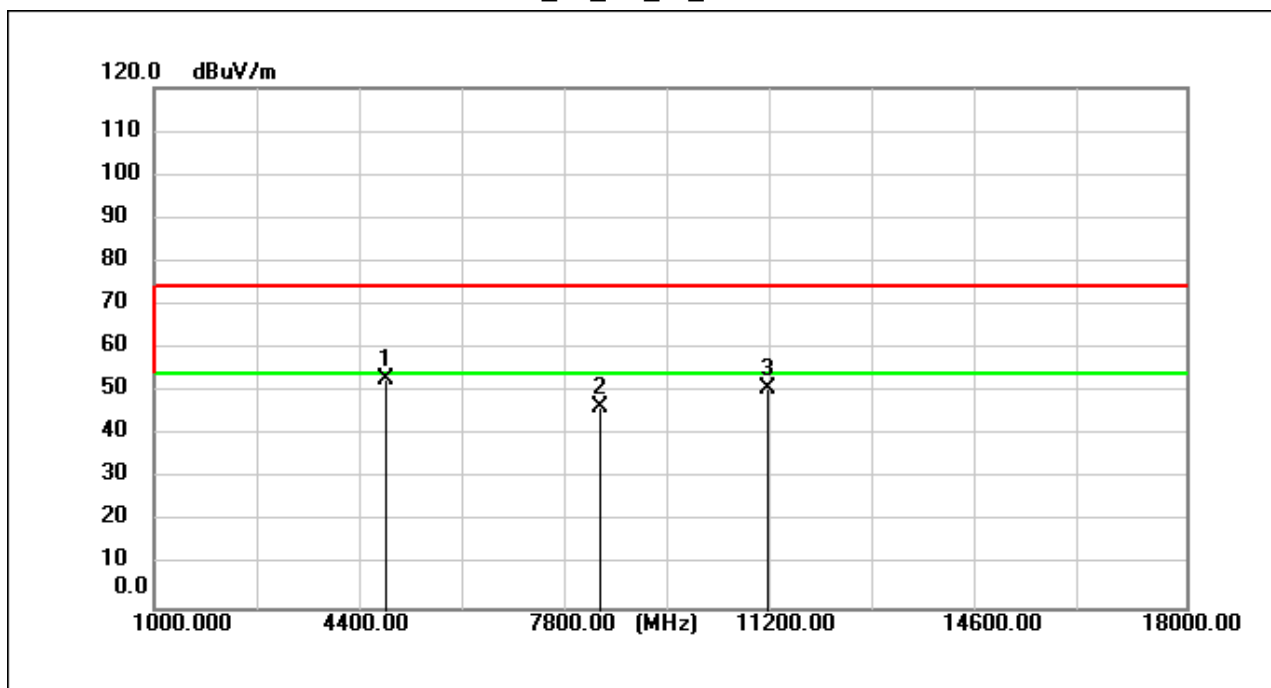
11b_TX_CH_01_Vertical
