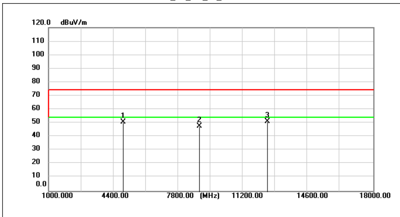
11b_TX_CH_11_Vertical
