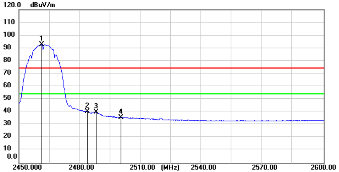
11b_TX_CH_11_Horizontal_Average
