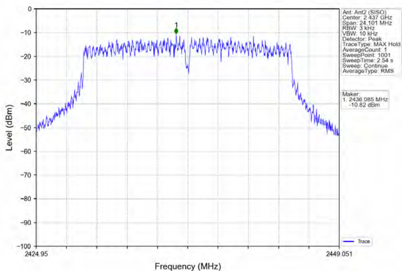
802.11g_MCH_2437MHz_Ant2 (SISO)_NTNV
