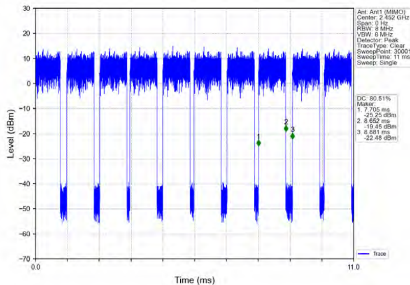
802.11n(HT40)_HCH_2452MHz_Ant1 (MIMO)_NTNV
