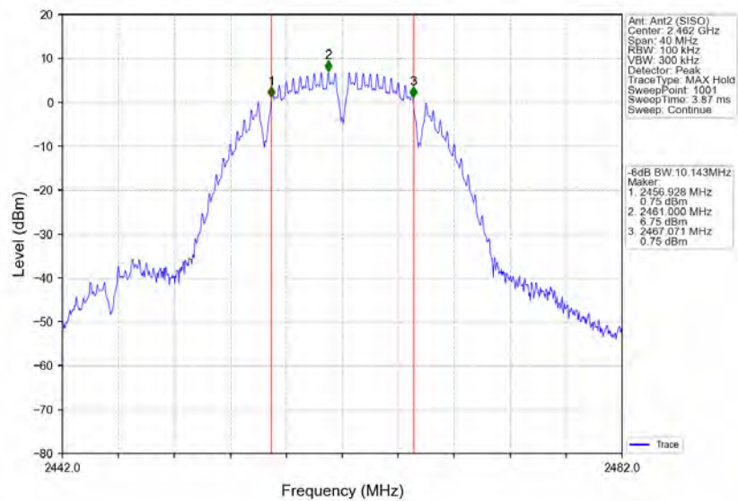
802.11b_HCH_2462MHz_Ant2 (SISO)_NTNV
