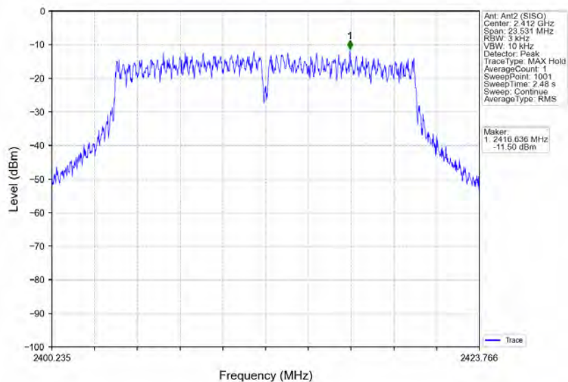
802.11g_LCH_2412MHz_Ant2 (SISO)_NTNV
