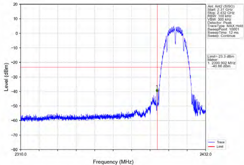
802.11b_LCH_2412MHz_Ant2 (SISO)_NTNV
