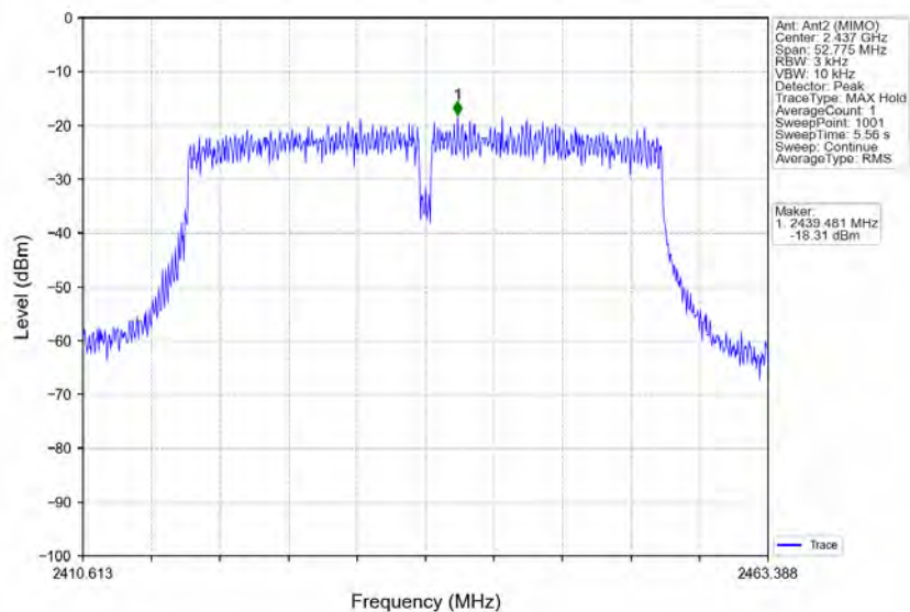
802.11n(HT40)_MCH_2437MHz_Ant2 (MIMO)_NTNV
