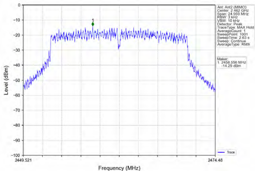
802.11n(HT20)_HCH_2462MHz_Ant2 (MIMO)_NTNV
