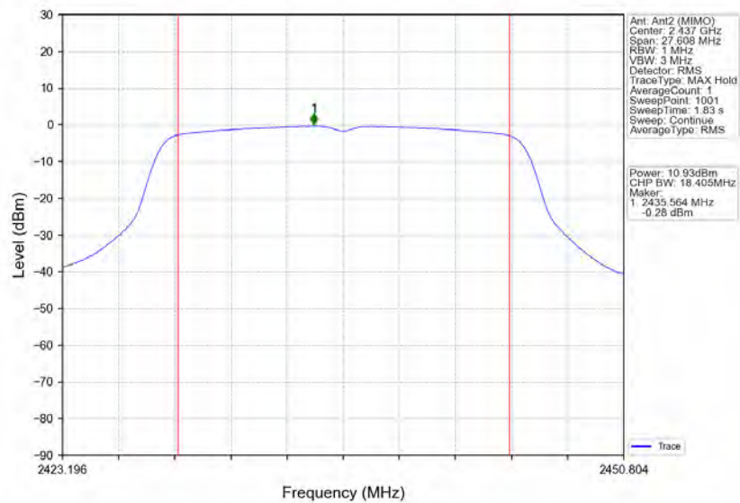
802.11n(HT20)_MCH_2437MHz_Ant2 (MIMO)_NTNV
