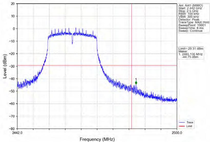
802.11n(HT20)_HCH_2462MHz_Ant1 (MIMO)_NTNV
