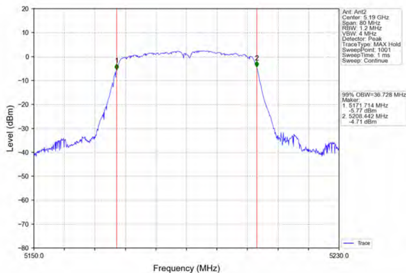
802.11n(HT40) LCH_5190MHz_Ant2_NTNV
