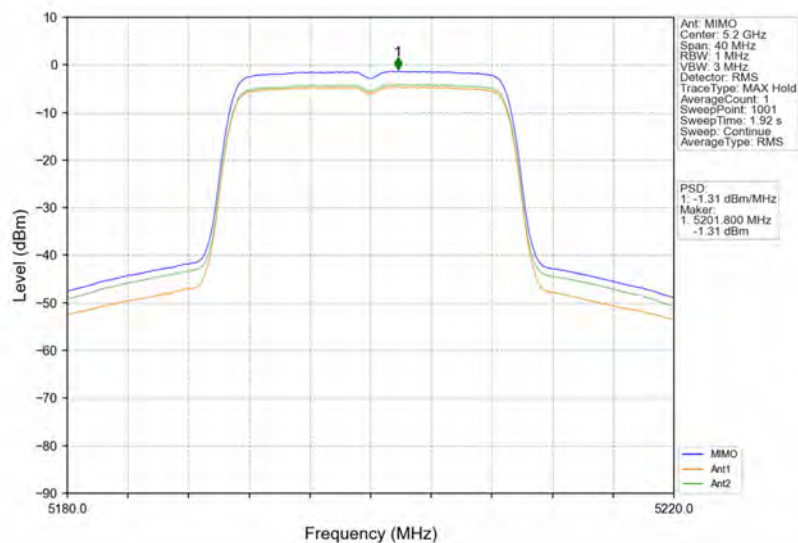
802.11n(HT20)_MCH_5200MHz_MIMO_NTNV
