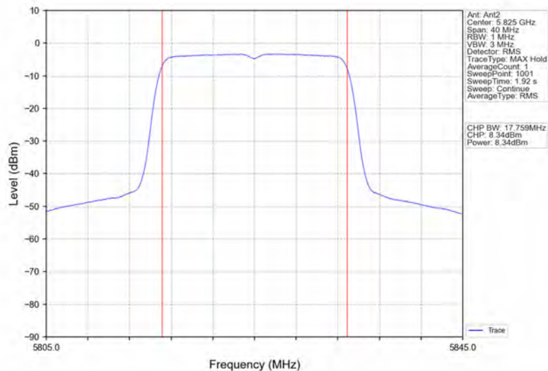
802.11n(HT20)_HCH_5825MHz_Ant2_NTNV
