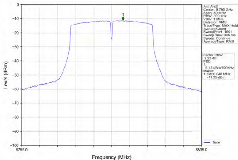
802.11n(HT40)_HCH_5795MHz_Ant2_NTNV
