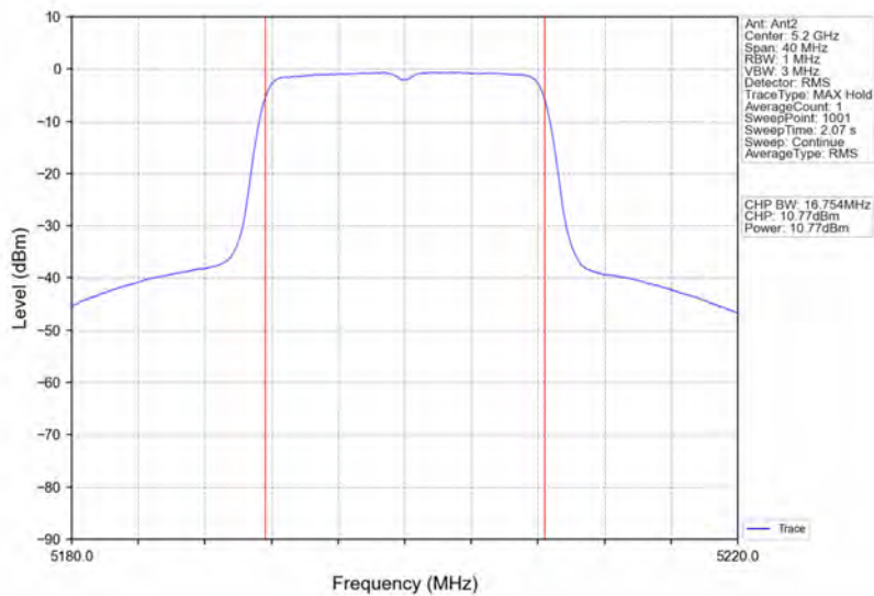
802.11a_MCH_5200MHz_Ant2_NTNV
