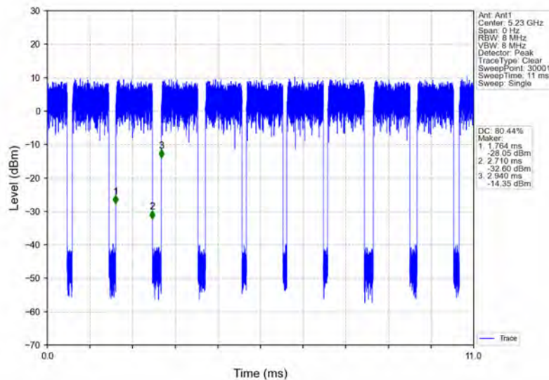
802.11n(HT40)_HCH_5230MHz_Ant1_NTNV
