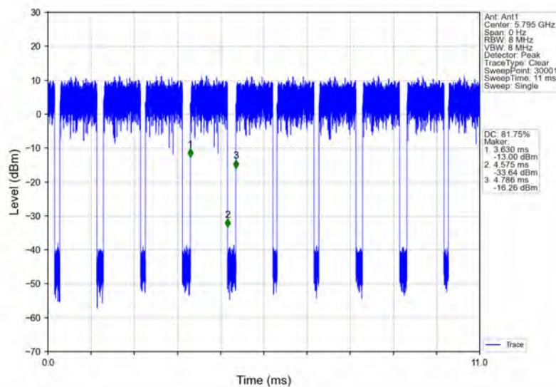
802.11n(HT40)_HCH_5795MHz_Ant1_NTNV
