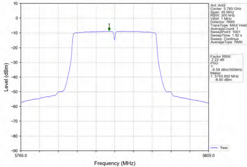
802.11n(HT20)_MCH_5785MHz_MIMO_NTNV
