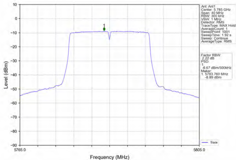
802.11n(HT20)_MCH_5785MHz_Ant1_NTNV
