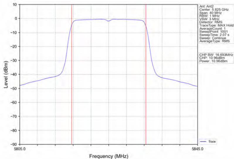
802.11a_HCH_5825MHz_Ant2_NTNV
