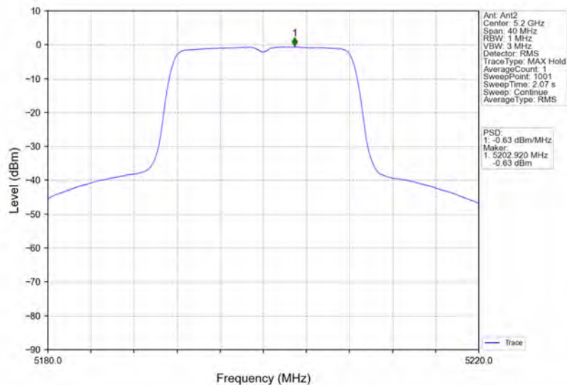
802.11a_MCH_5200MHz_Ant2_NTNV
