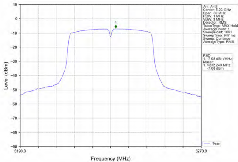
802.11n(HT40)_HCH_5230MHz_Ant2_NTNV
