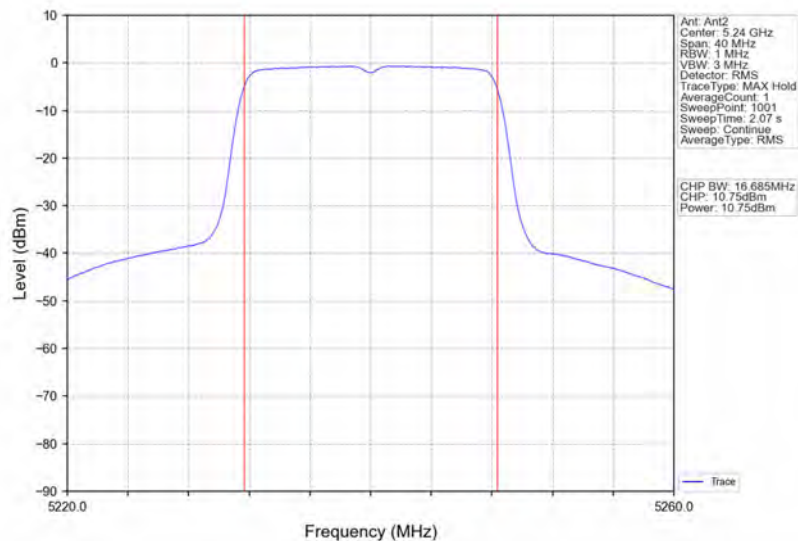
802.11a_HCH_5240MHz_Ant2_NTNV
