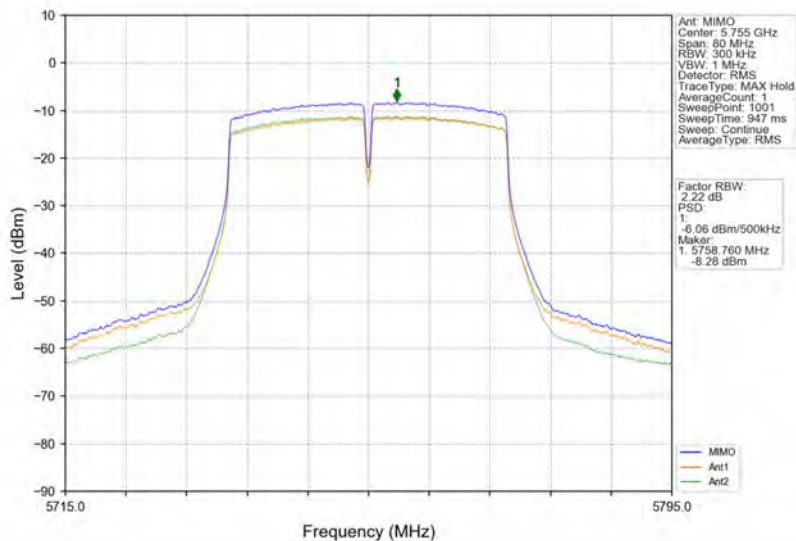
802.11n(HT40)_LCH_5755MHz_MIMO_NTNV
