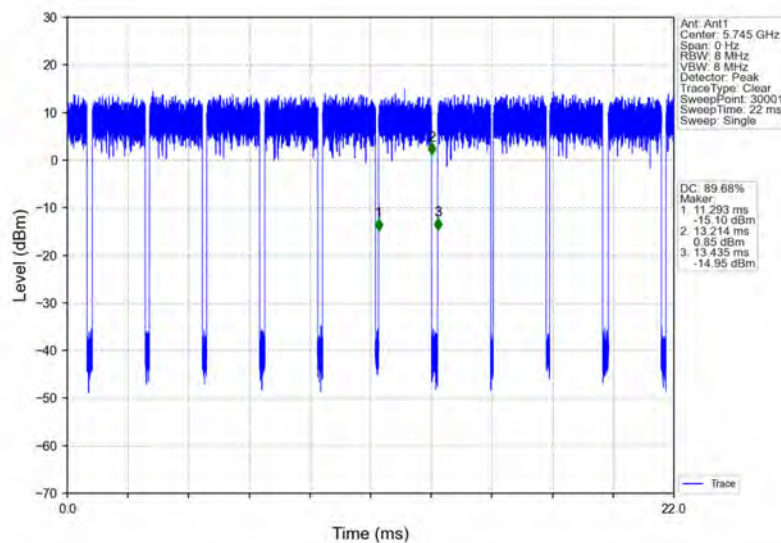
802.11n(HT20)_LCH_5745MHz_Ant1_NTNV
