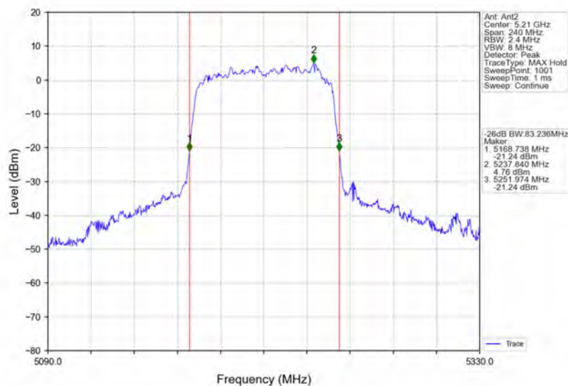
802.11ac(VHT80)_MCH_5210MHz_Ant2_NTNV
