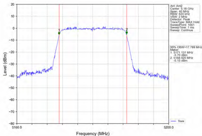
802.11n(HT20)_LCH_5180MHz_Ant2_NTNV
