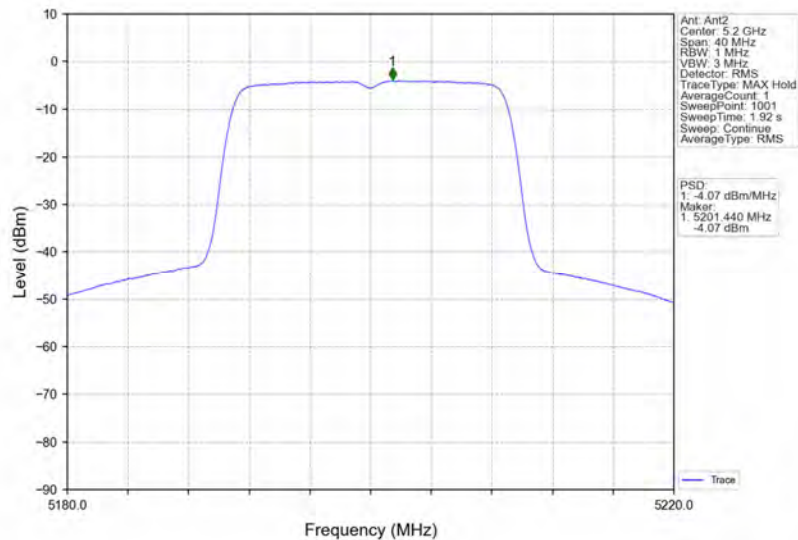
802.11n(HT20)_MCH_5200MHz_MIMO_NTNV
