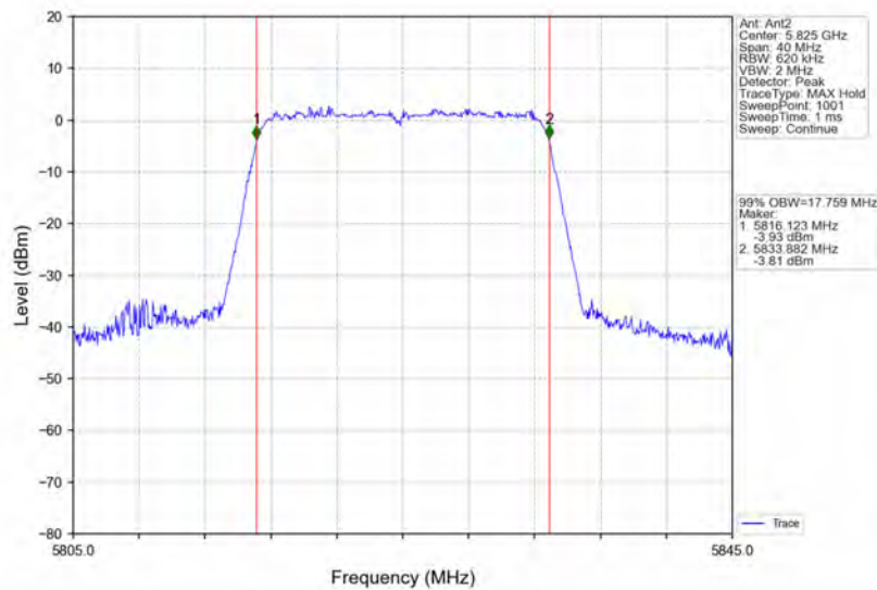
802.11n(HT20)_HCH_5825MHz_Ant2_NTNV
