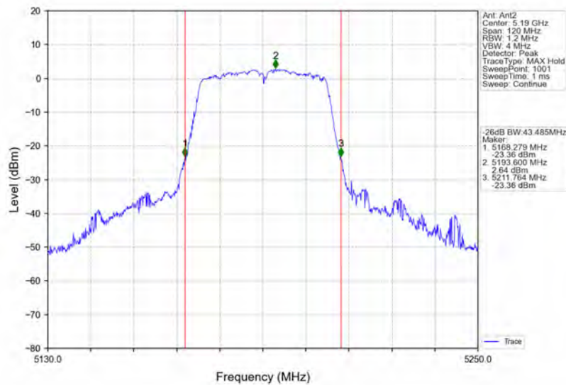
802.11n(HT40)_LCH_5190MHz_Ant2_NTNV
