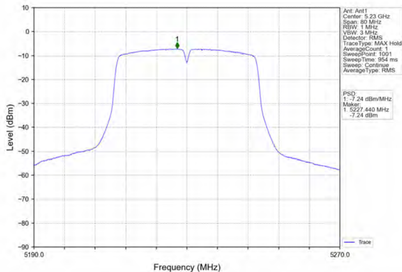
802.11ac(VHT40)_HCH_5230MHz_Ant1_NTNV
