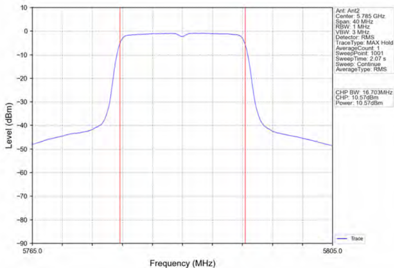
802.11a_MCH_5785MHz_Ant2_NTNV
