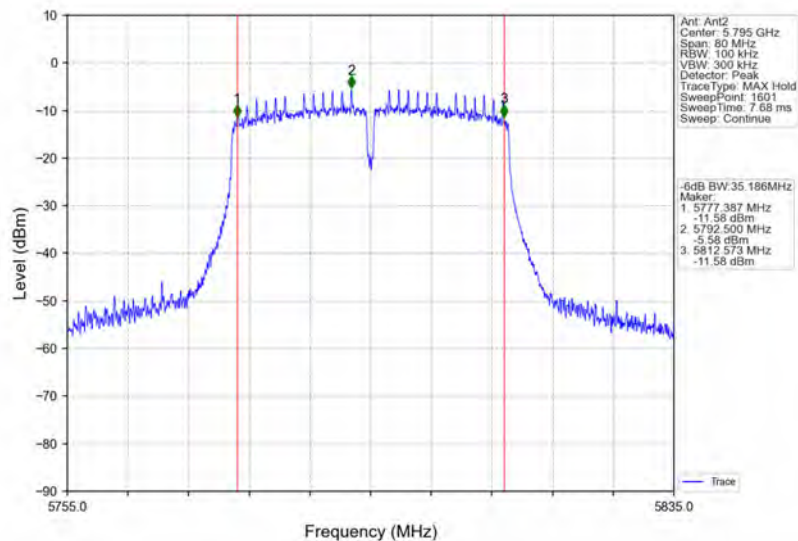
802.11n(HT40)_HCH_5795MHz_Ant2_NTNV
