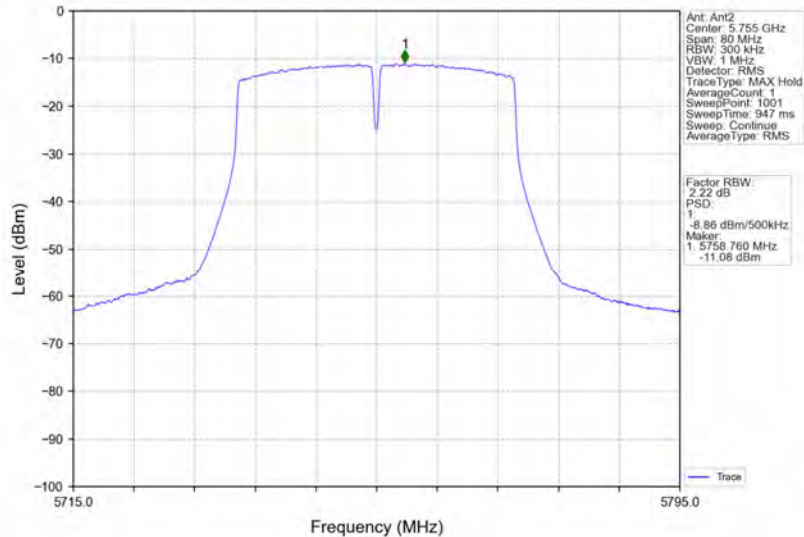
802.11n(HT40)_LCH_5755MHz_MIMO_NTNV
