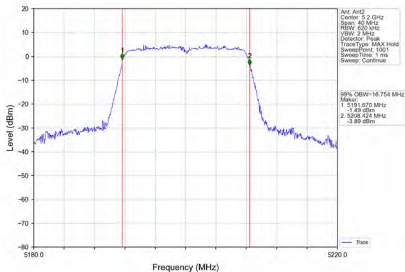
802.11a_MCH_5200MHz_Ant2_NTNV
