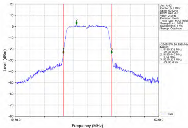
802.11n(HT20)_MCH_5200MHz_Ant2_NTNV
