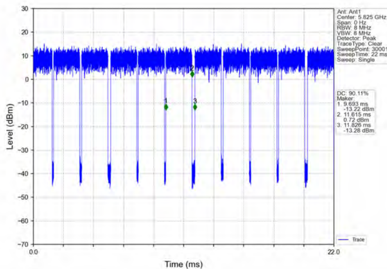
802.11n(HT20)_HCH_5825MHz_Ant1_NTNV
