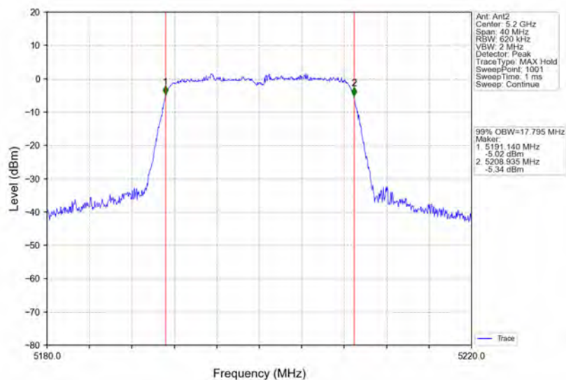
802.11n(HT20)_MCH_5200MHz_Ant2_NTNV
