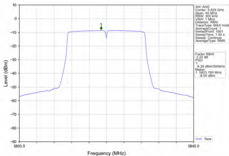
802.11n(HT20)_HCH_5825MHz_Ant2_NTNV
