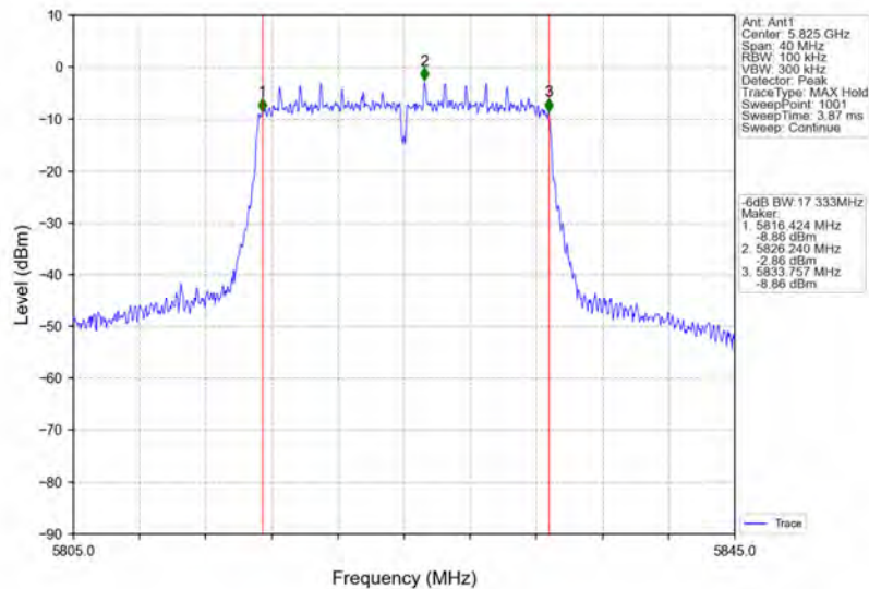
802.11n(HT20)_HCH_5825MHz_Ant2_NTNV
