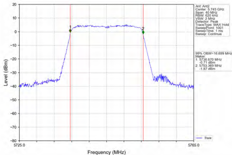
802.11a_LCH_5745MHz_Ant2_NTNV
