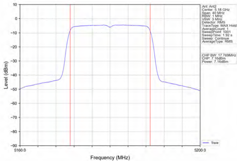
802.11n(HT20)_LCH_5180MHz_Ant2_NTNV
