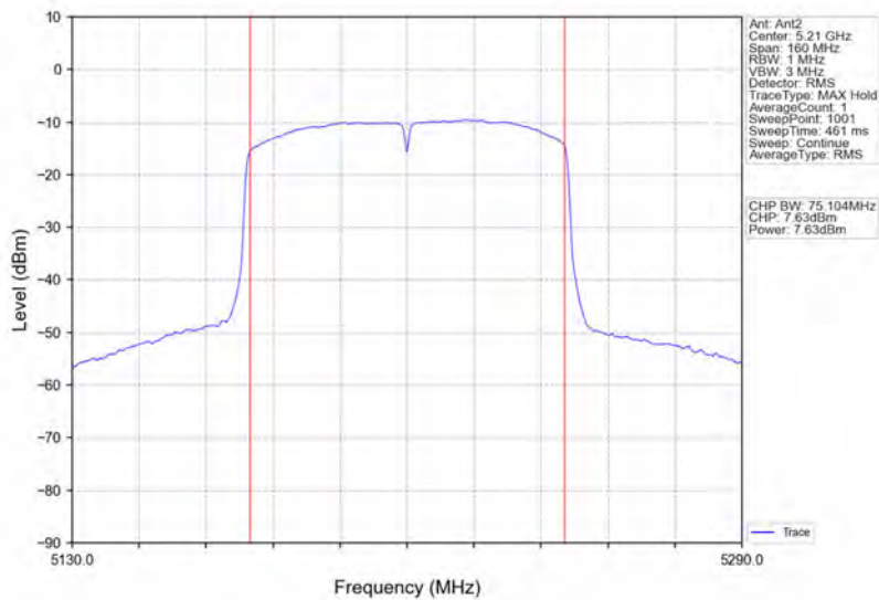
802.11ac(VHT80)_MCH_5210MHz_Ant2_NTNV
