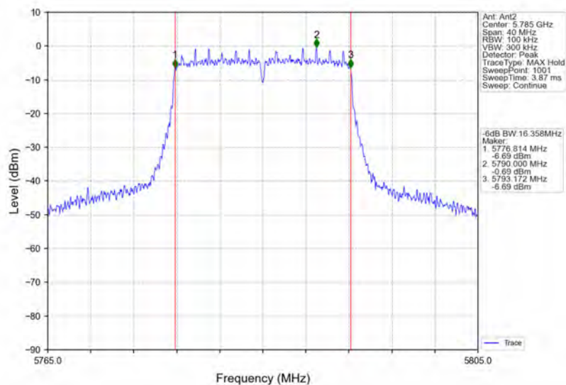
802.11a_MCH_5785MHz_Ant2_NTNV
