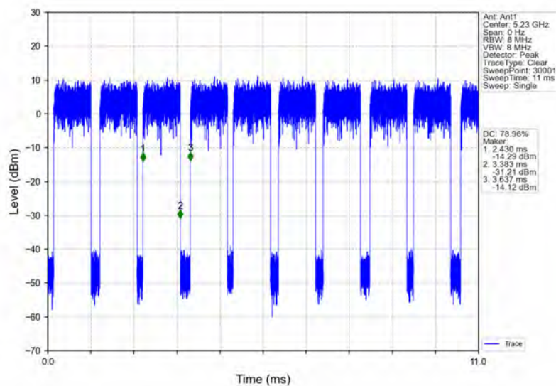
802.11ac(VHT40)_HCH_5230MHz_Ant1_NTNV
