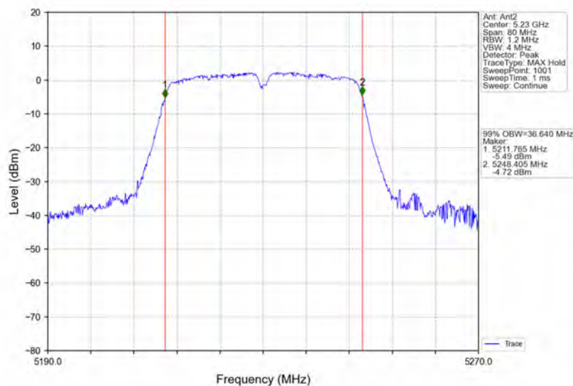
802.11n(HT40)_HCH_5230MHz_Ant2_NTNV
