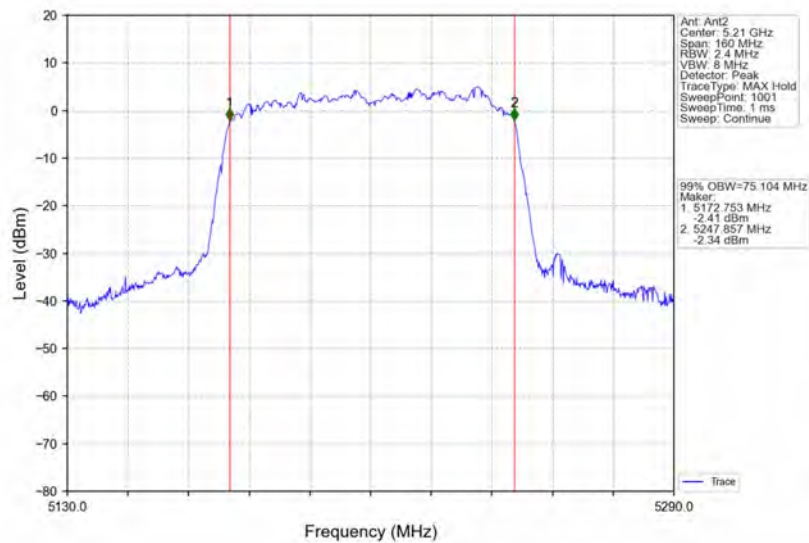
802.11ac(VHT80)_MCH_5210MHz_Ant2_NTNV
