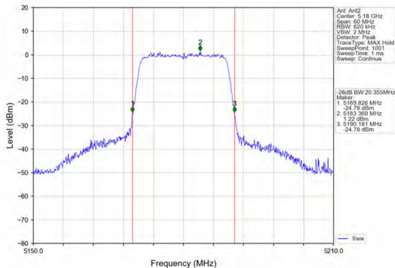
802.11n(HT20)_LCH_5180MHz_Ant2_NTNV
