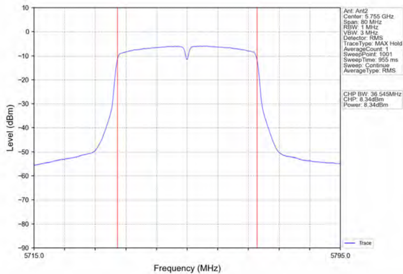
802.11ac(VHT40)_LCH_5755MHz_Ant2_NTNV
