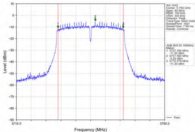
802.11ac(VHT40)_LCH_5755MHz_Ant2_NTNV
