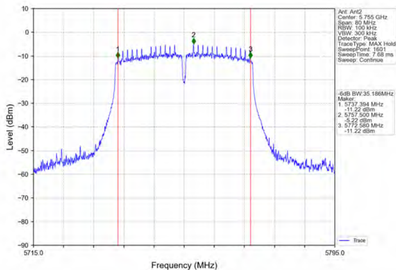
802.11n(HT40) LCH_5755MHz_Ant2_NTNV
