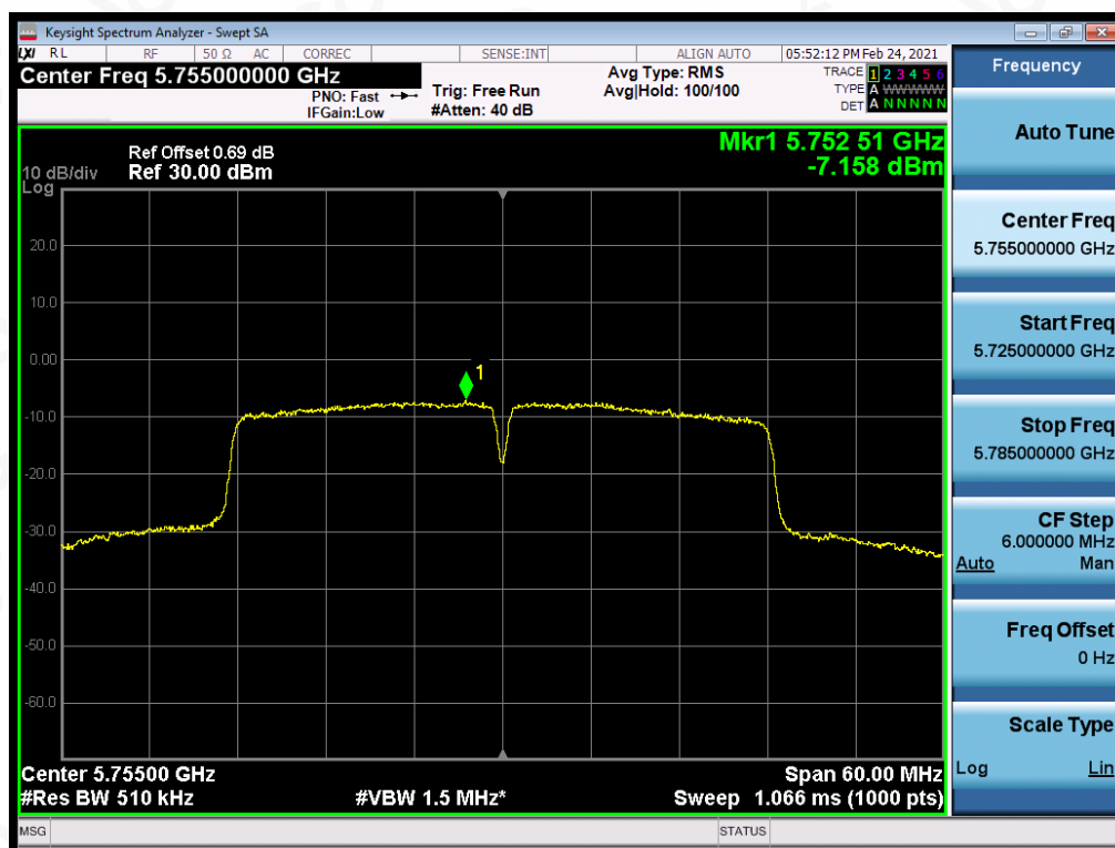
Test Graph 802.11n40 ANT1 5755 MCS0 PSD
