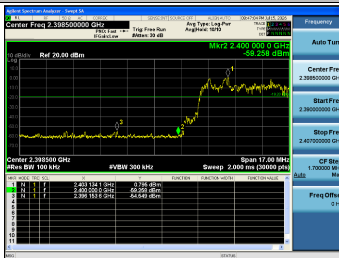
2DH5_Ant1_Hop_Low
