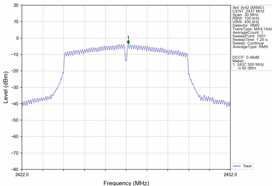
802.11n(HT20)_MCH_2437MHz_MIMO_NTNV
