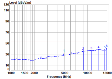
11n_40M_TX_CH_09_Horizontal-Avg
