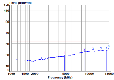
11n_40M_TX_CH_06_Vertical-Avg
