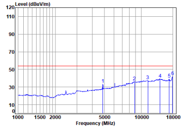
11n_40M_TX_CH_06_Horizontal-Avg
