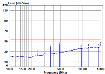
11b_TX_CH_06_Vertical-Avg
