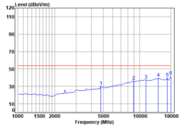
11n_40M_TX_CH_03_Vertical-Avg
