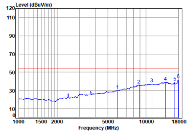
11n_40M_TX_CH_09_Vertical-Avg
