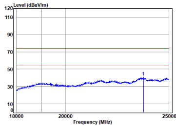
11b_TX_CH_01_Vertical
