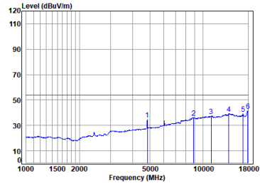
11n_40M_TX_CH_03_Horizontal-Avg
