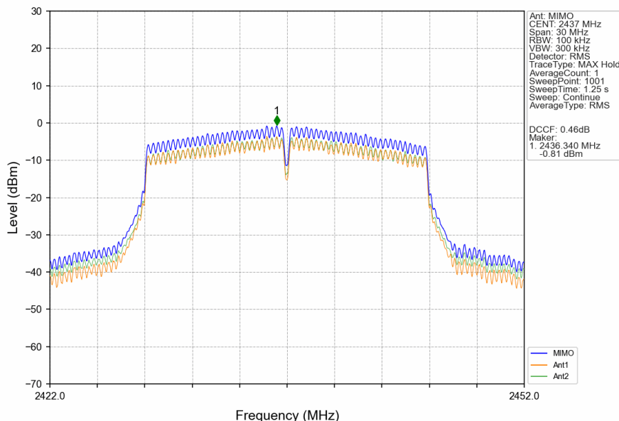
802.11n(HT20)_MCH_2437MHz_MIMO_NTNV
