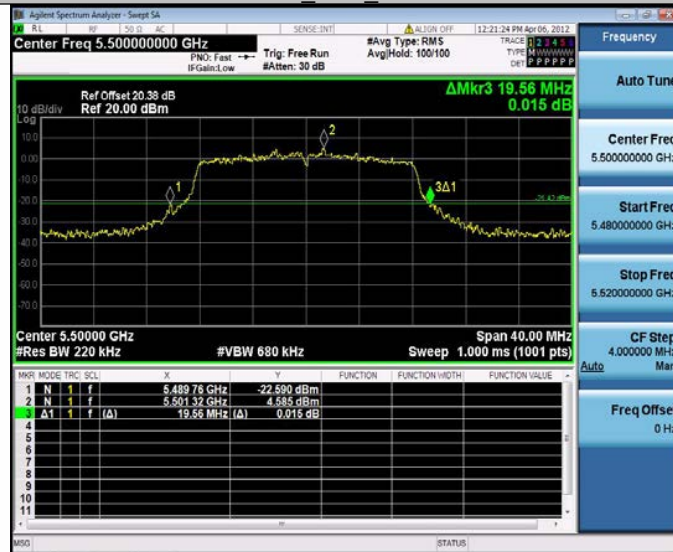
11A_Ant4_5500
