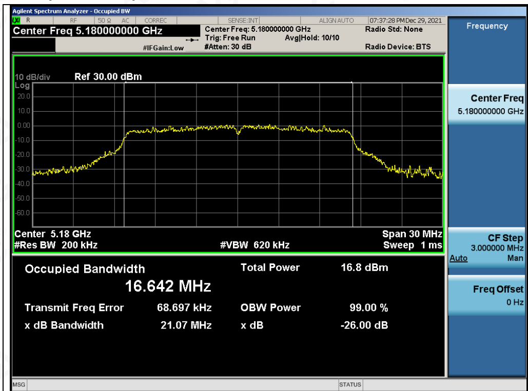
Test_Graph_802.11a_ANT1_5180_6Mbps_OBW
