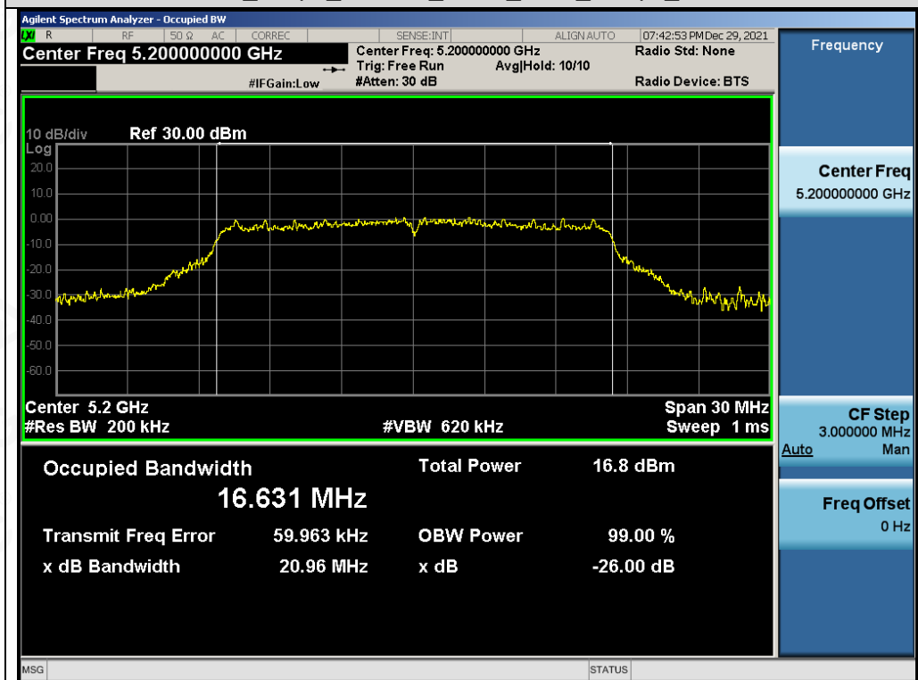
Test_Graph_802.11a_ANT1_5200_6Mbps_OBW
