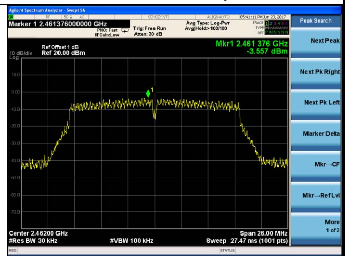
PSD - CH 11 - 802.11g
