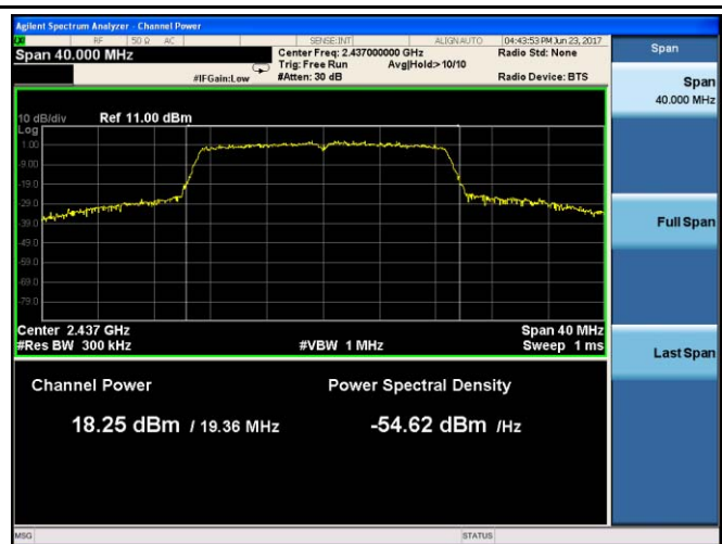
802.11n20 - AV Output power - CH 6
