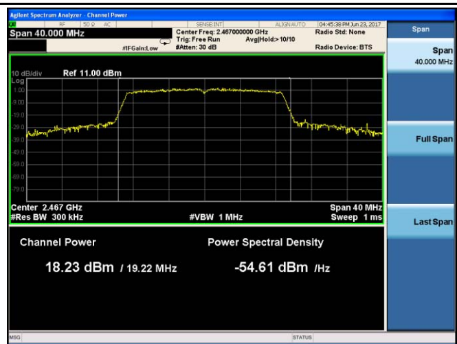
802.11n20 - AV Output power - CH 12
