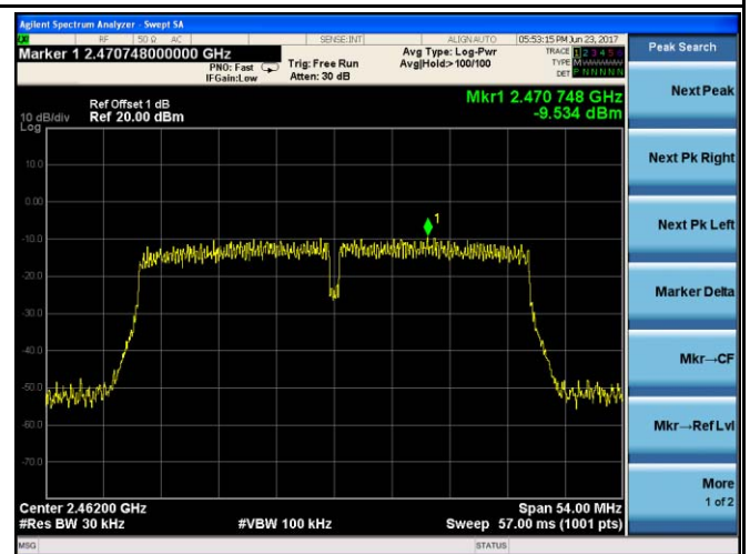
PSD - CH 11 - 802.11n40
