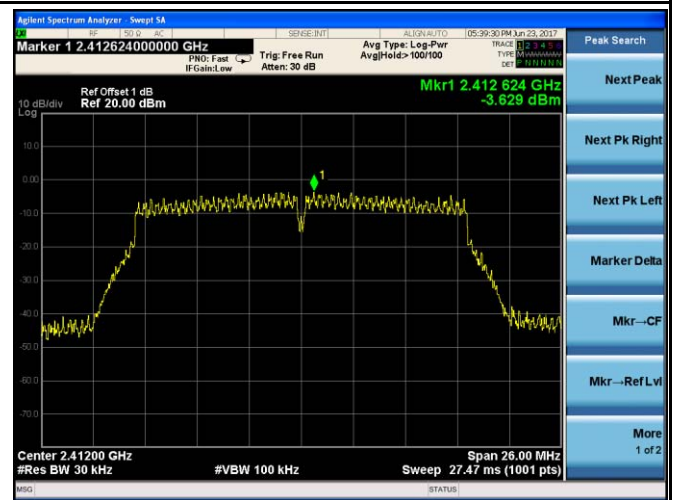
PSD - CH 1 - 802.11g
