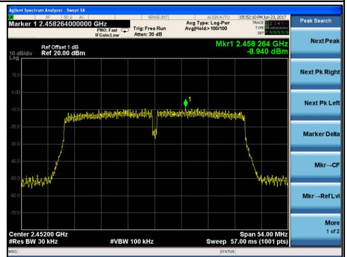
PSD - CH 9 - 802.11n40
