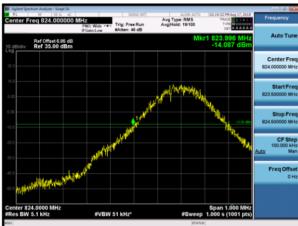
GSM 850-LCH-EDGE
