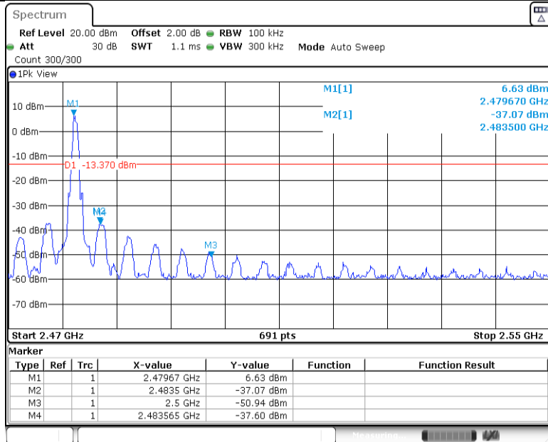
BLE BT5.0 Ant1 High 2480 MHz
