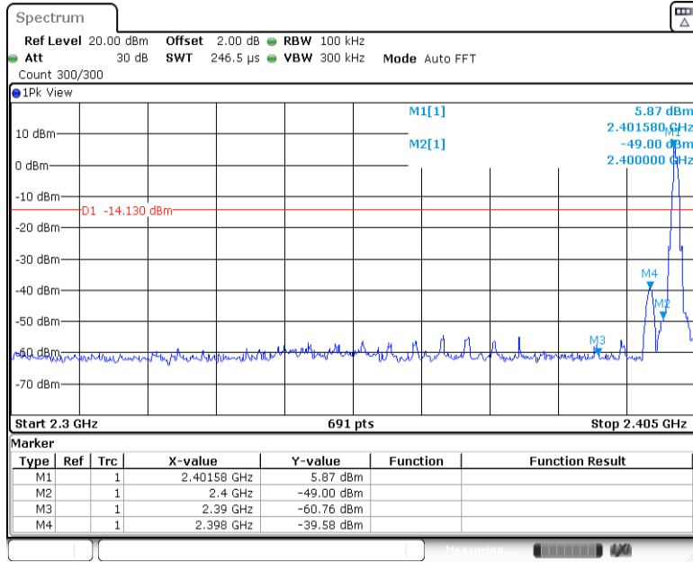
BLE BT5.0 Ant1 Low 2402 MHz
