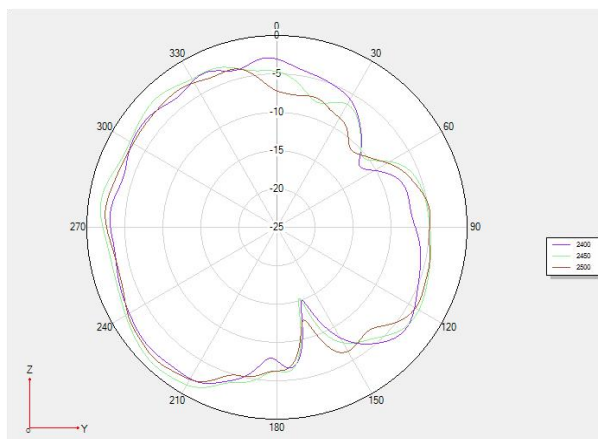
Phi 90 2D图
