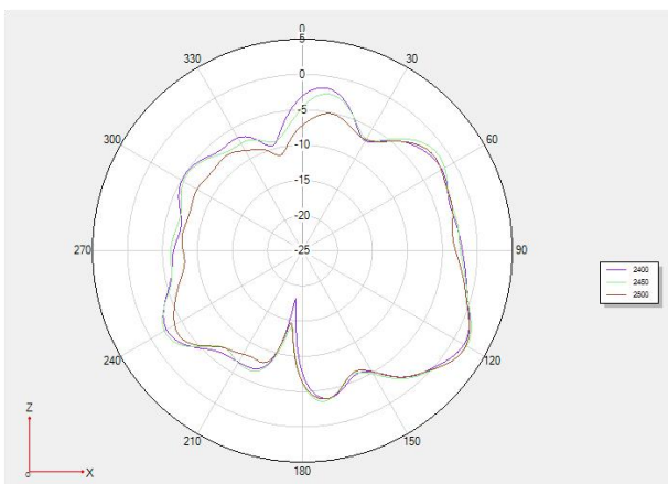
Phi 0 2D图
