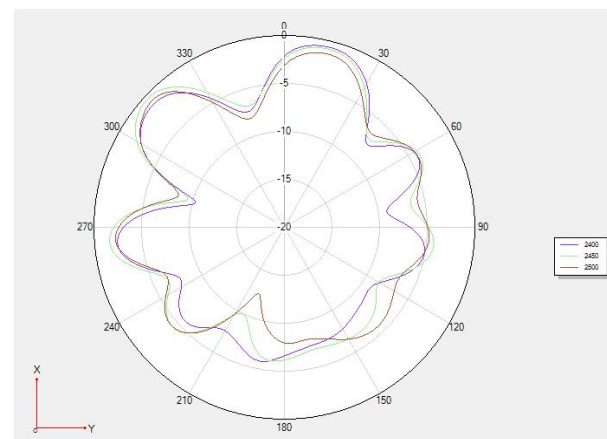
Theta 90 2D图
