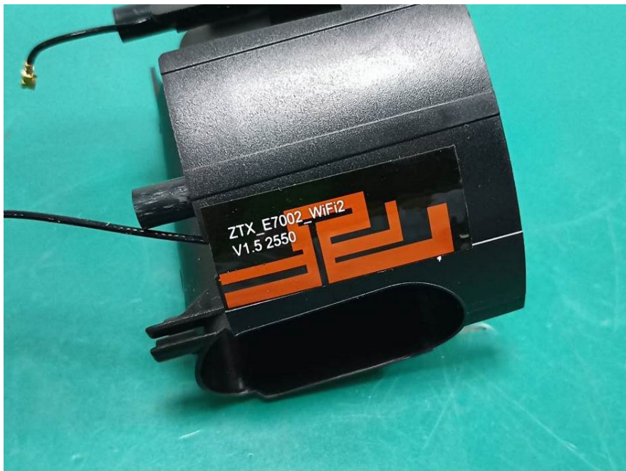
Wi-Fi ANT 1
