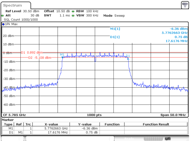
802.11ac20_5785MHz_Chain 0
