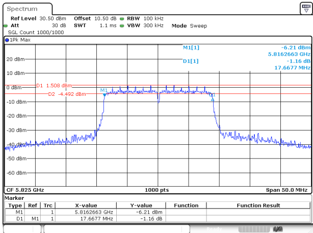
802.11ac20_5825MHz_Chain 0
