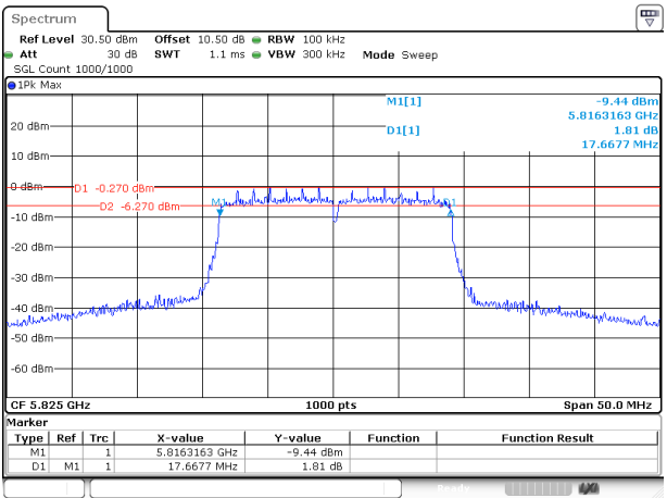
802.11ac20_5825MHz_Chain 1
