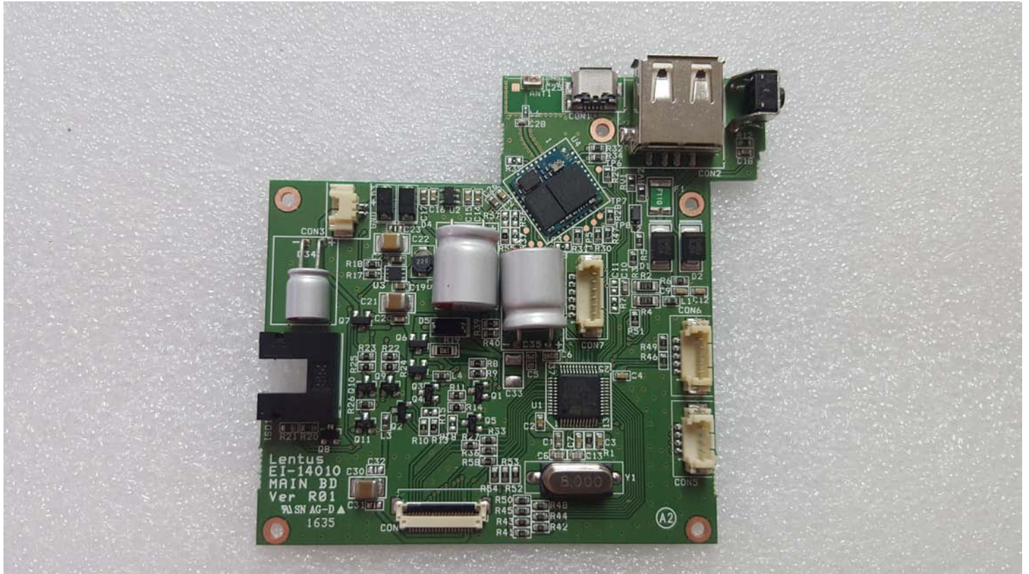
MainBoard_Front.jpg (5312 X 2988)
