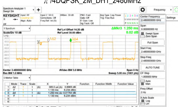
\pi /4DQPSK_2M_DH1_2480MHz
