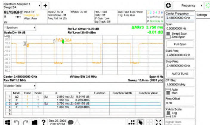
\pi /4DQPSK_2M_DH5_2480MHz
