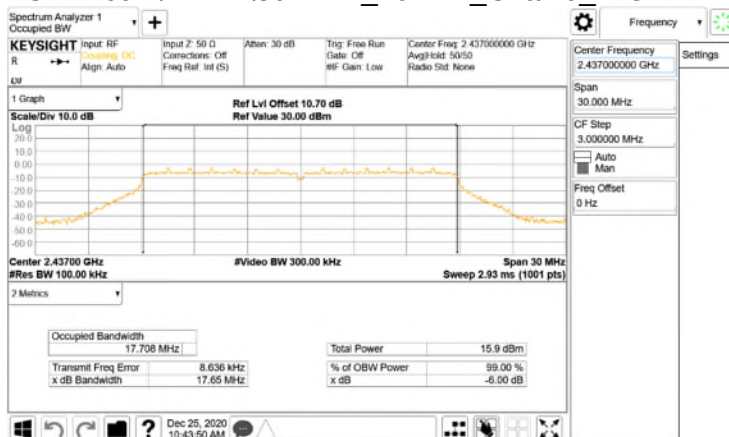
OBW 6dBWLAN\802.11n_20MHz_Chain0_2437MHz
