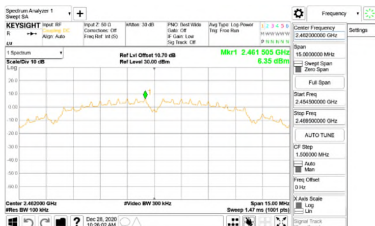
Reference Level\WLAN\802.11b_20MHz_Chain0_2462MHz
