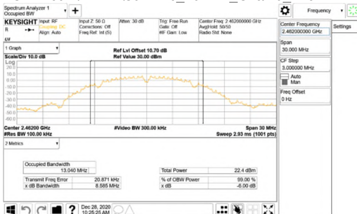
OBW 6dBWLAN\802.11b_20MHz_Chain0_2462MHz
