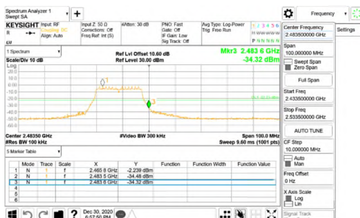
Band Edge\WLAN\802.11n_20MHz_Chain0_2472MHz
