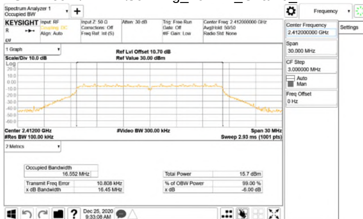
OBW 6dBWLAN\802.11g_20MHz_Chain0_2412MHz
