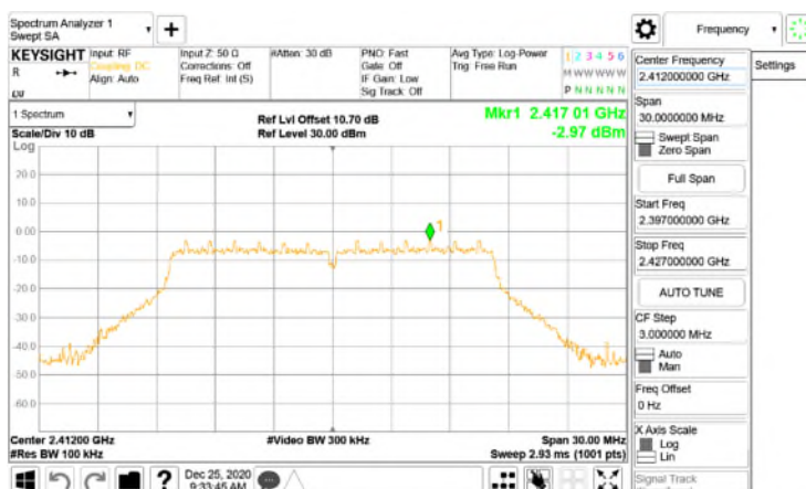
Reference Level\WLAN\802.11g_20MHz_Chain0_2412MHz
