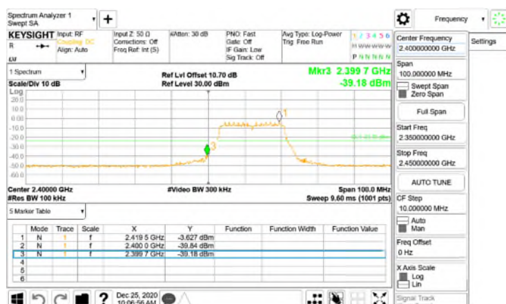
Band Edge\WLAN\802.11n_20MHz_Chain0_2412MHz
