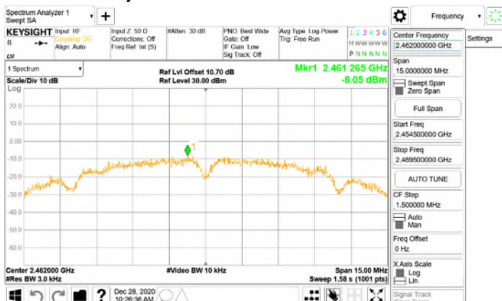
Power Density\WLAN\802.11b_20MHz_Chain0_2462MHz
