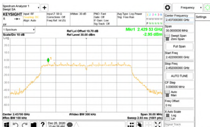
Reference Level\WLAN\802.11n_20MHz_Chain0_2437MHz
