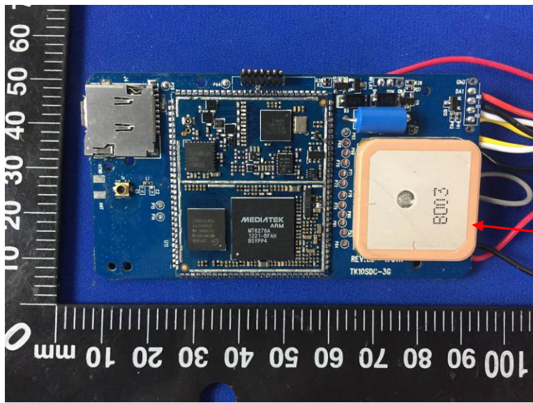
GPS Antenna
