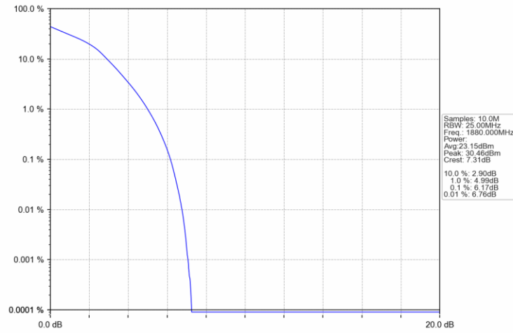
Band2 20MHz 16QAM MCH 1880MHz RB 100 0 NTNV
