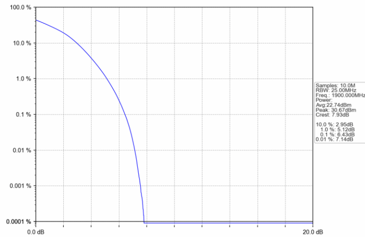
Band2 20MHz 16QAM HCH 1900MHz RB 100 0 NTNV
