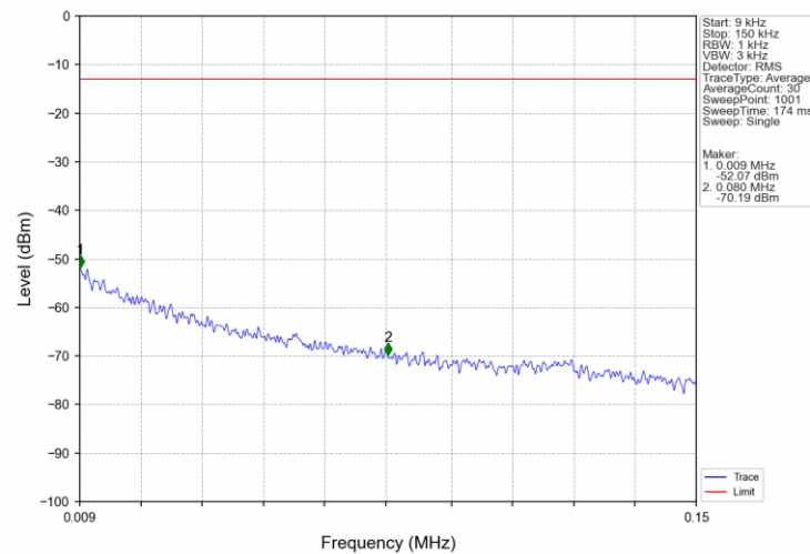
Band2 1.4MHz 16QAM HCH 1909.3MHz RB 1 0 NTV
