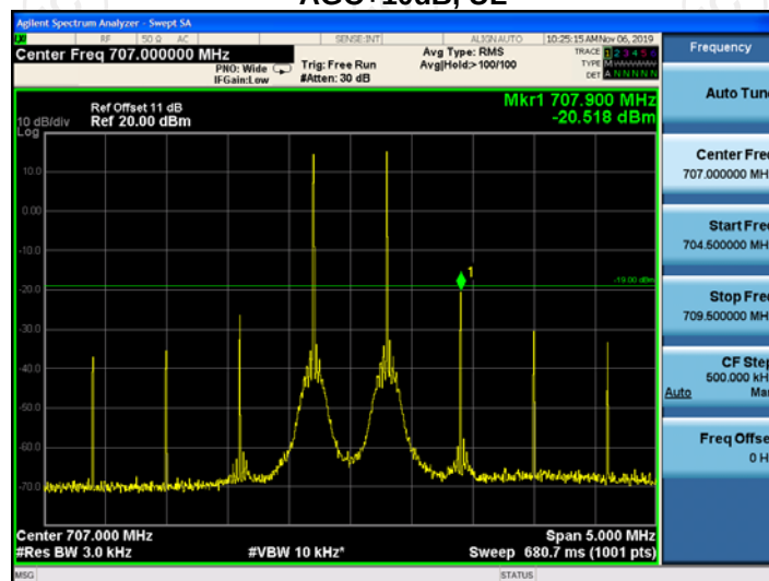
AGC+10dB, UL
