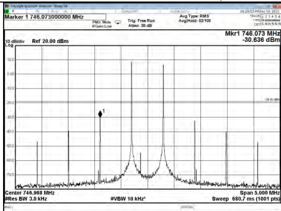
Upper 700MHz band Pre AGC, DL
