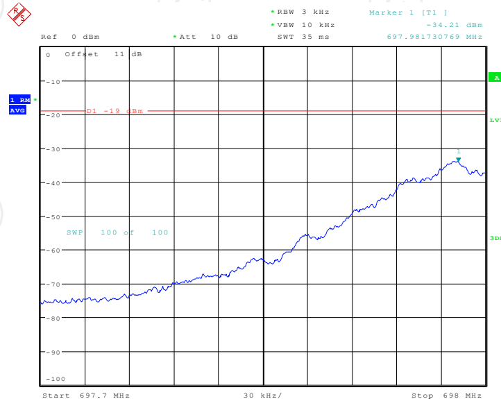
Lower700MHz GSM UL Left Side Pre AGC+10dB
