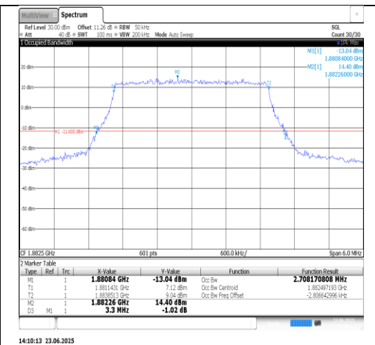
Band25-5MHz-QPSK-26365-25RB#0-PASS
