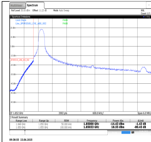
Band2-5MHz-QPSK-18625-25RB#0-PASS
