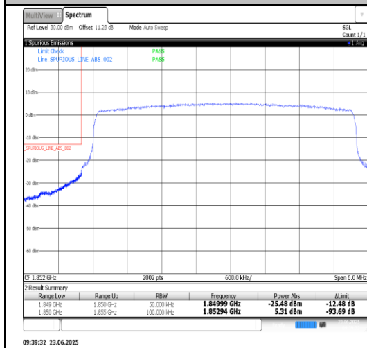
Band2-5MHz-QPSK-18625-25RB#24-PASS
