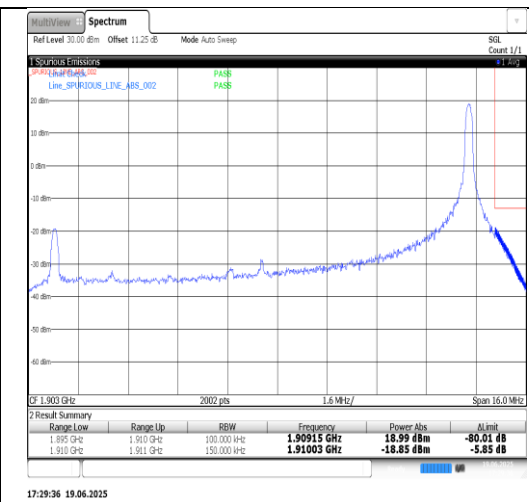
Band2-20MHz-QPSK-18700-1RB#99-PASS
