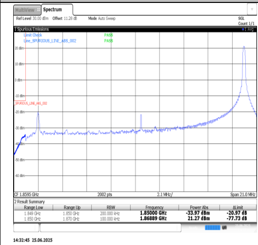
Band2-20MHz-QPSK-18700-100RB#99-PASS
