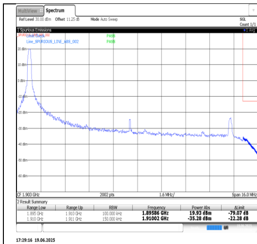
Band2-20MHz-QPSK-18700-1RB#0-PASS
