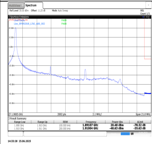
Band2-20MHz-QPSK-19100-1RB#99-PASS
