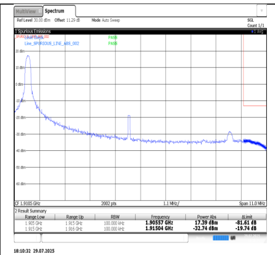
Band25-10MHz-QPSK-26640-50RB#0-PASS
