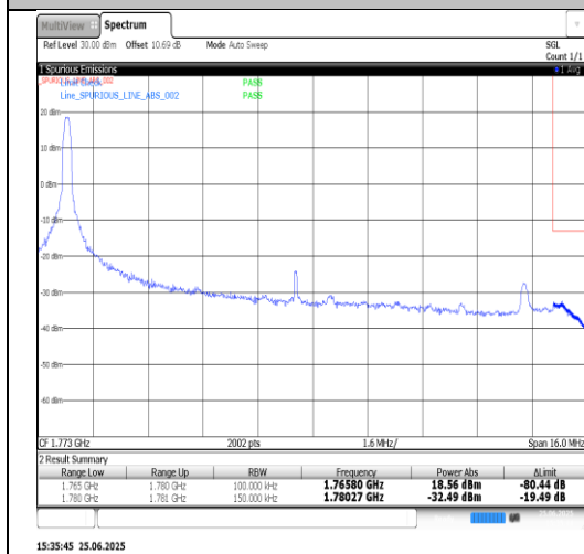
Band66-20MHz-QPSK-132072-1RB#0-PASS
