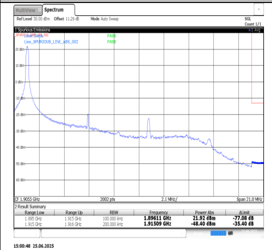
Band25-20MHz-QPSK-26590-100RB#0-PASS
