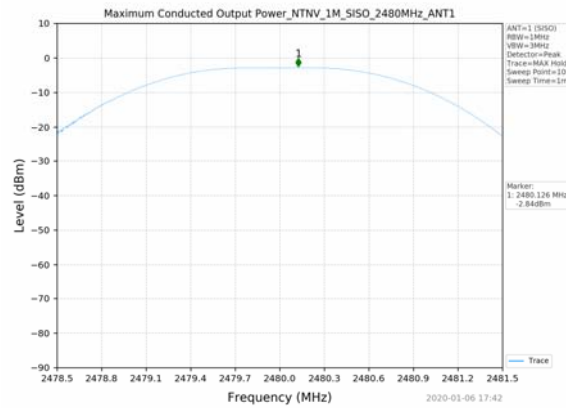
1M_2480MHz_SISO_ANT1
