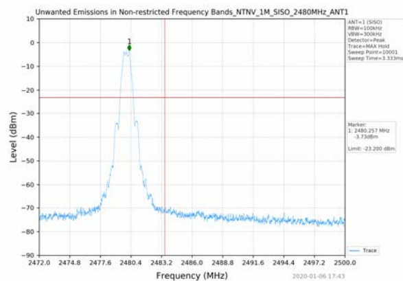
1M_2480MHz_SISO_ANT1
