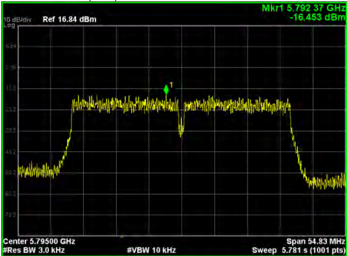
802.11ac40 channel 159(mimo)
