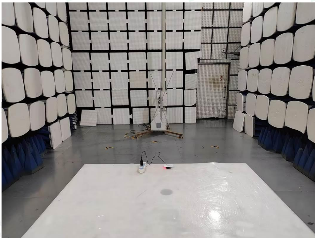
Fig. 2 (30MHz~1GHz)
