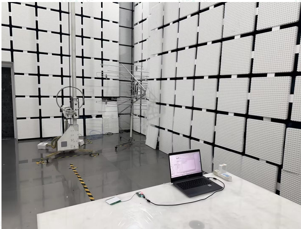
Fig. 1 (Below 30MHz)
