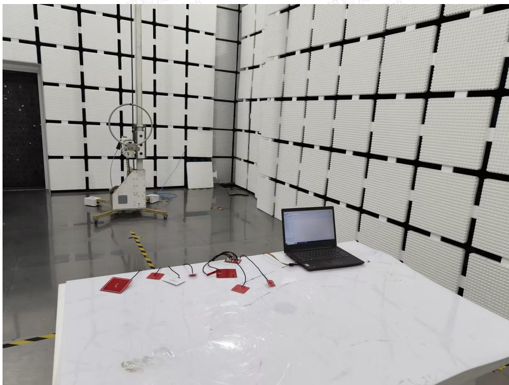
Fig. 3 (Below 30MHz)
