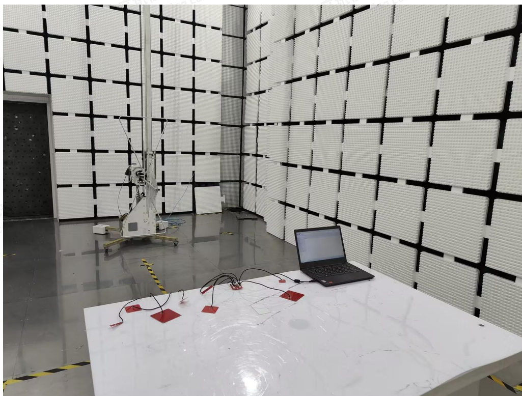
Fig. 6 (30MHz~1GHz)
