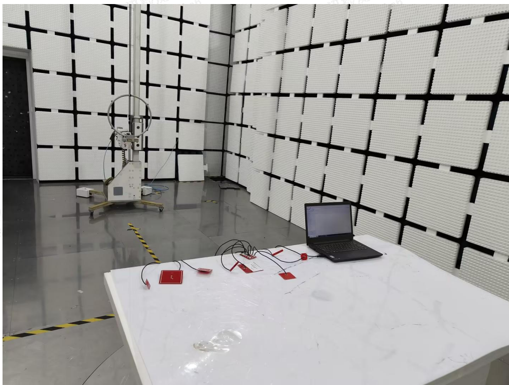
Fig. 5 (Below 30MHz)
