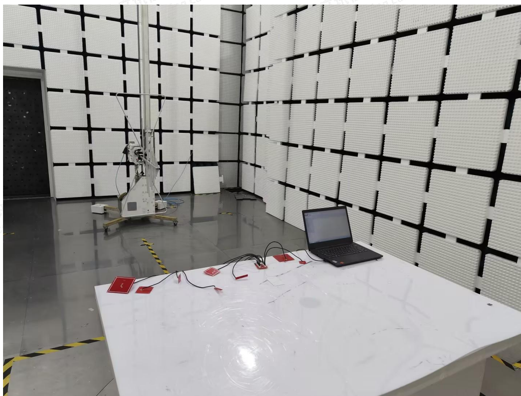
Fig. 8 (30MHz~1GHz)
