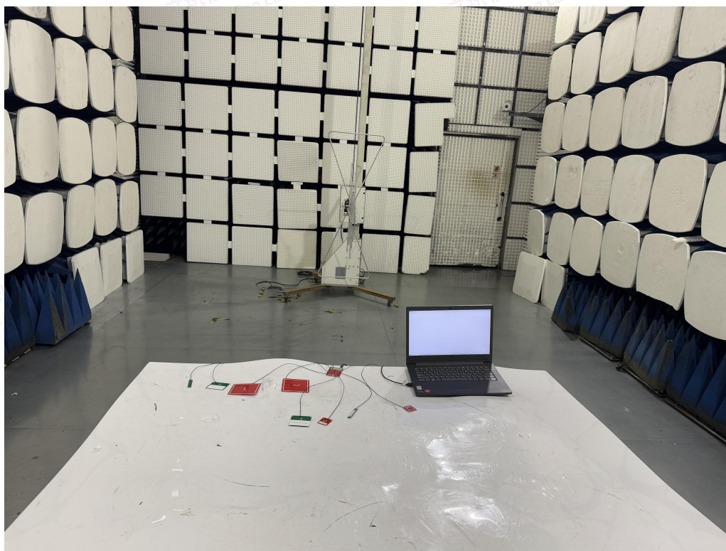
Fig. 8 (30MHz~1GHz)
