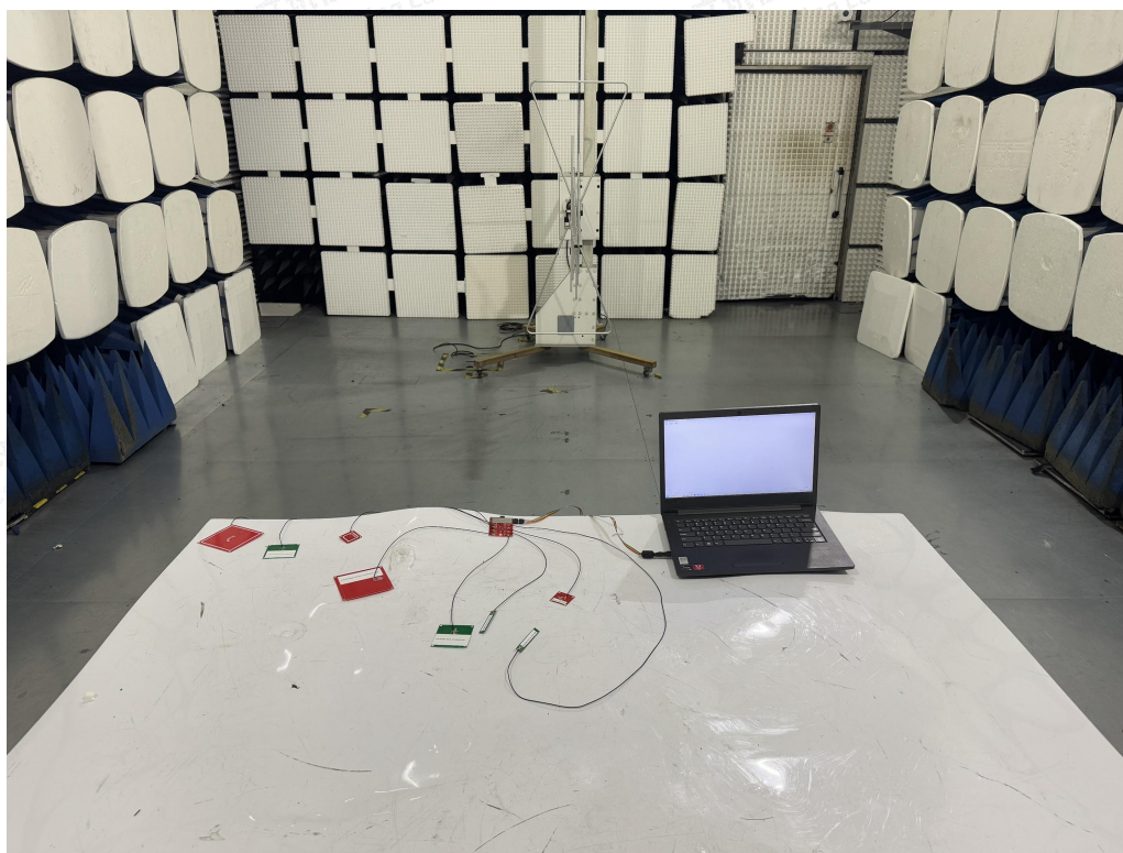
Fig. 4 (30MHz~1GHz)
