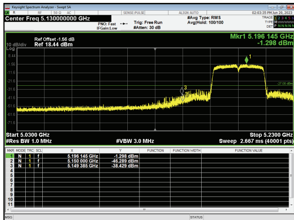
Band Edge n20 5180MHz Low
