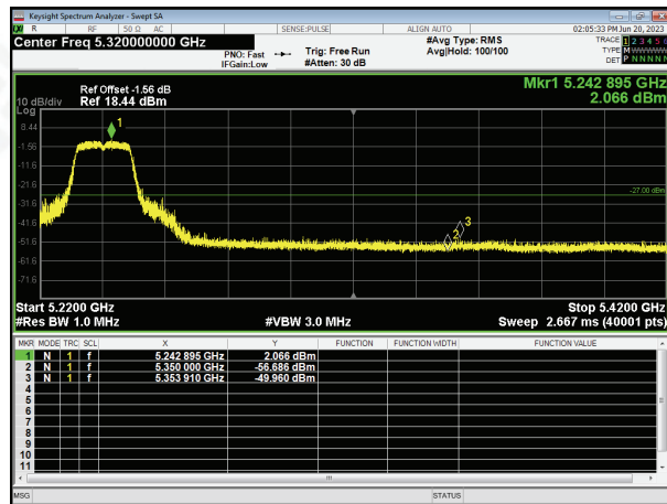
Band Edge ac40 5230MHz High
