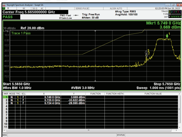
Band Edge ac20 5745MHz
