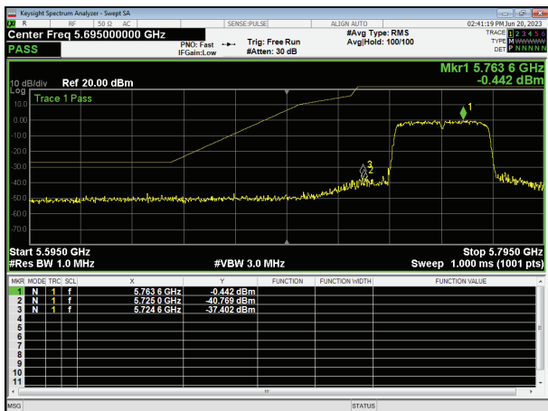
Band Edge n40 5755MHz
