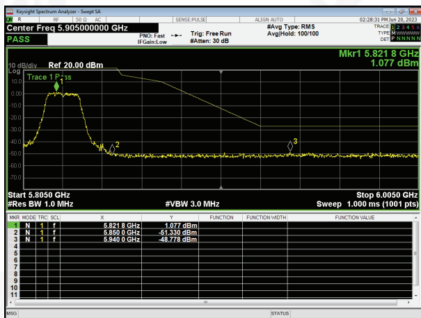
Band Edge ac20 5825MHz
