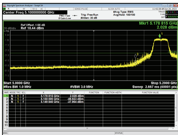
Band Edge ac20 5180MHz Low
