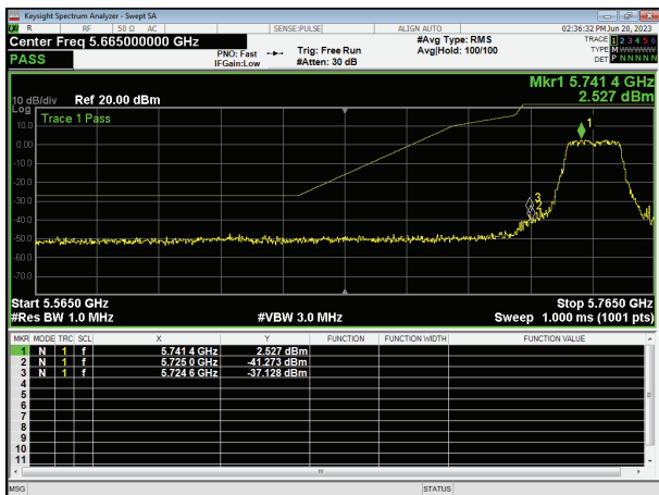
Band Edge ac40 5755MHz
