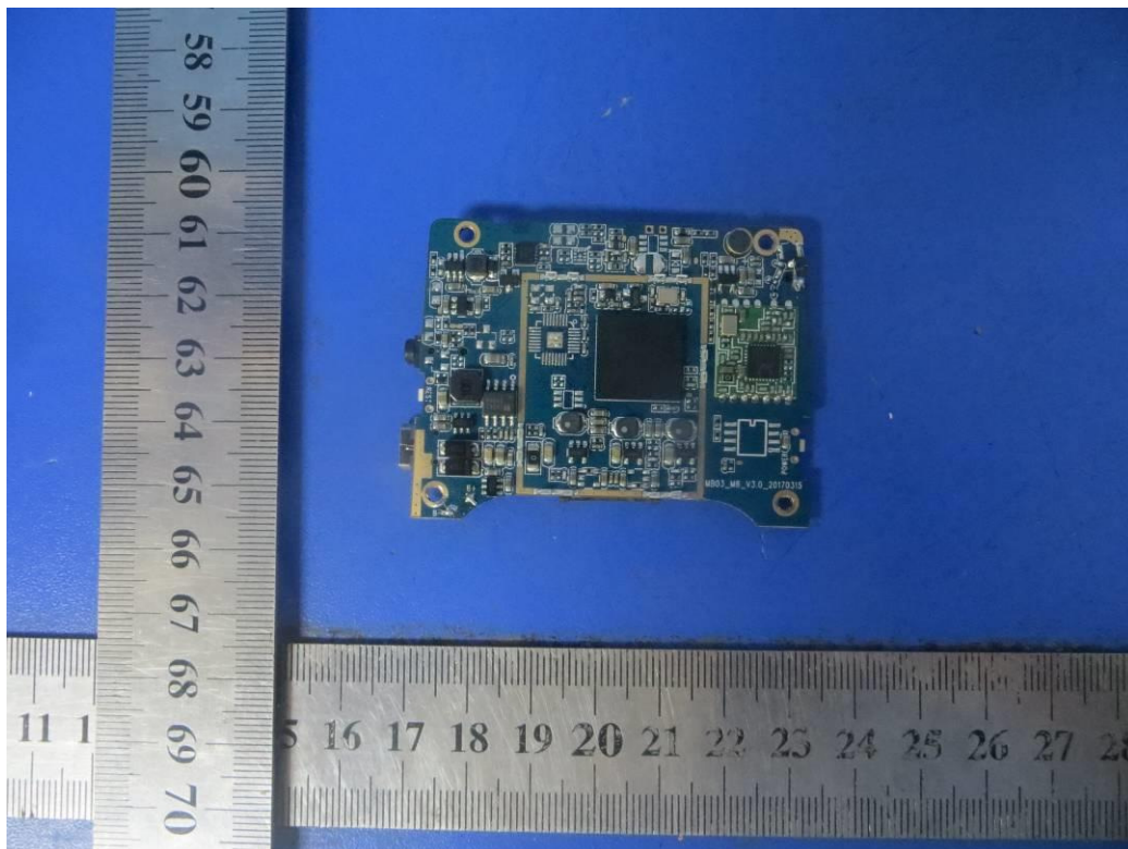
Fig.7 A307_PCB _Front
