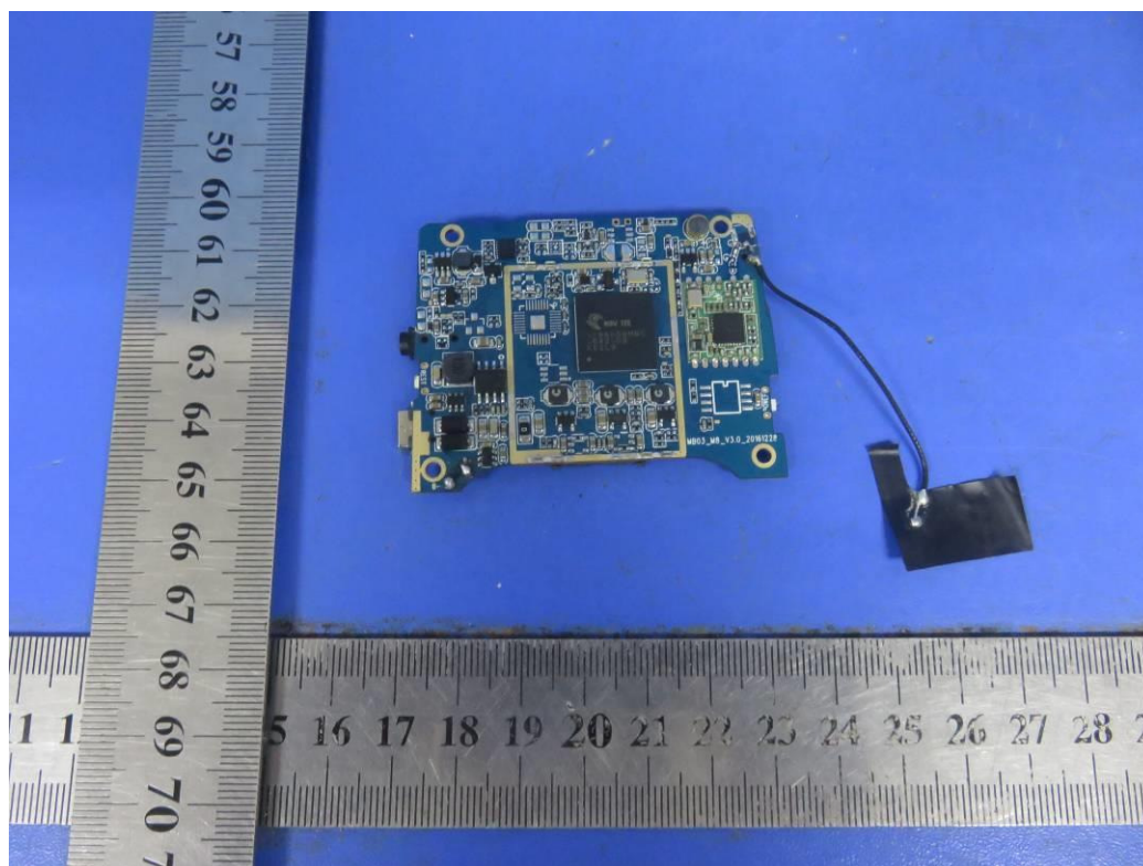
Fig.2 A305_PCB_Front
